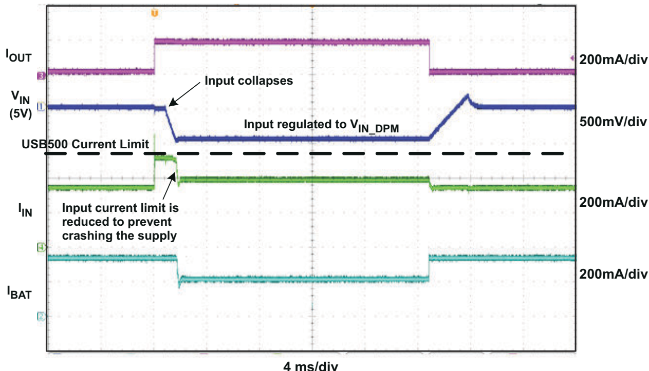
图 9-3. V_{IN\_DPM} Waveform
