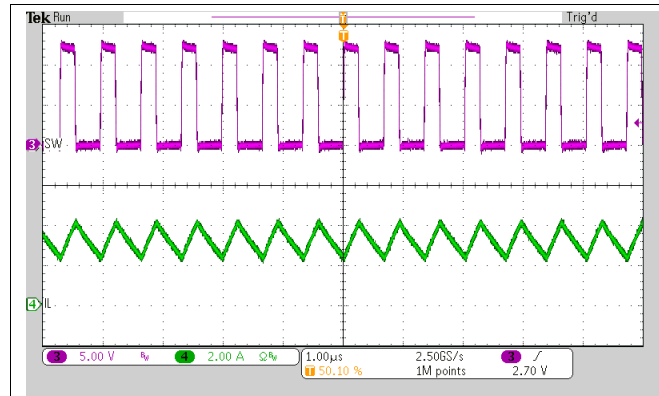
图 26. PWM Switching in Buck mode
