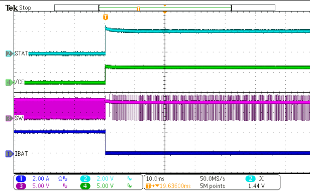
图 26. PWM Switching in Buck mode
