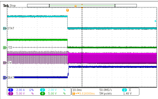
图 9-10. Charge Enable
