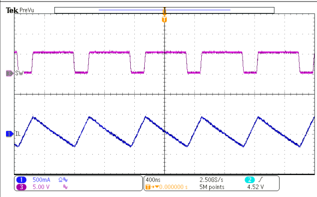
图 9-12. OTG Switching
