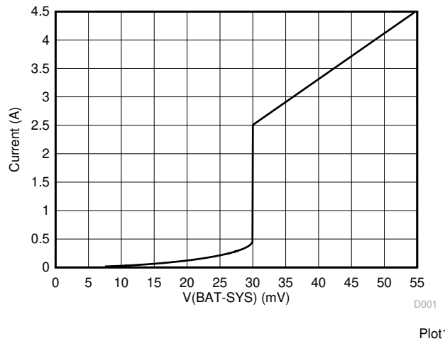
图 8-9. BAFET V-I Curve
