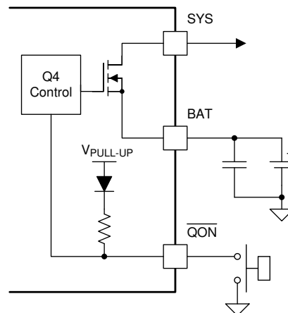
图 9-11. \overline{QON} Circuit
