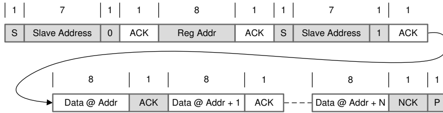
图 9-19. Multi-Read
