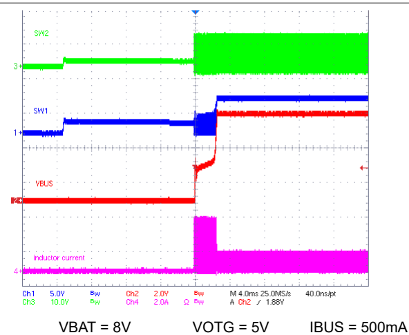
图 9-6. OTG Startup at 500-mA Load
