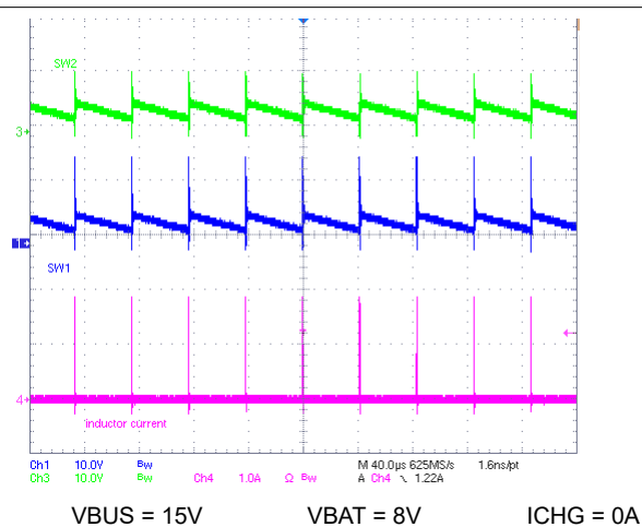
图 9-3. Buck Mode PFM with OOA
