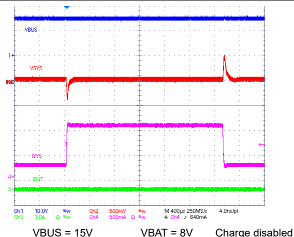
图 9-7. VSYS Load Transient Response
