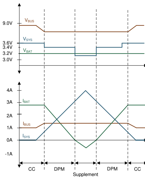
图 8-9. DPM Response
