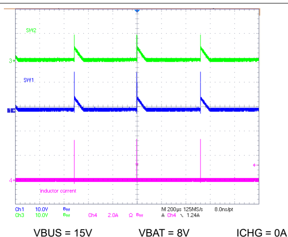
图 9-4. Buck Mode PFM without OOA
