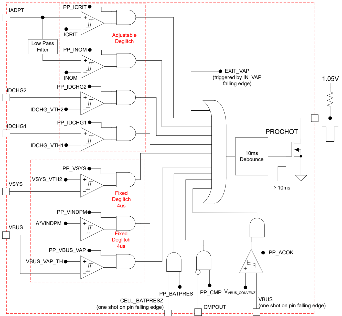
图 9-4. PROCHOT Profile
