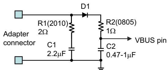
图 10-2. Input Filter
