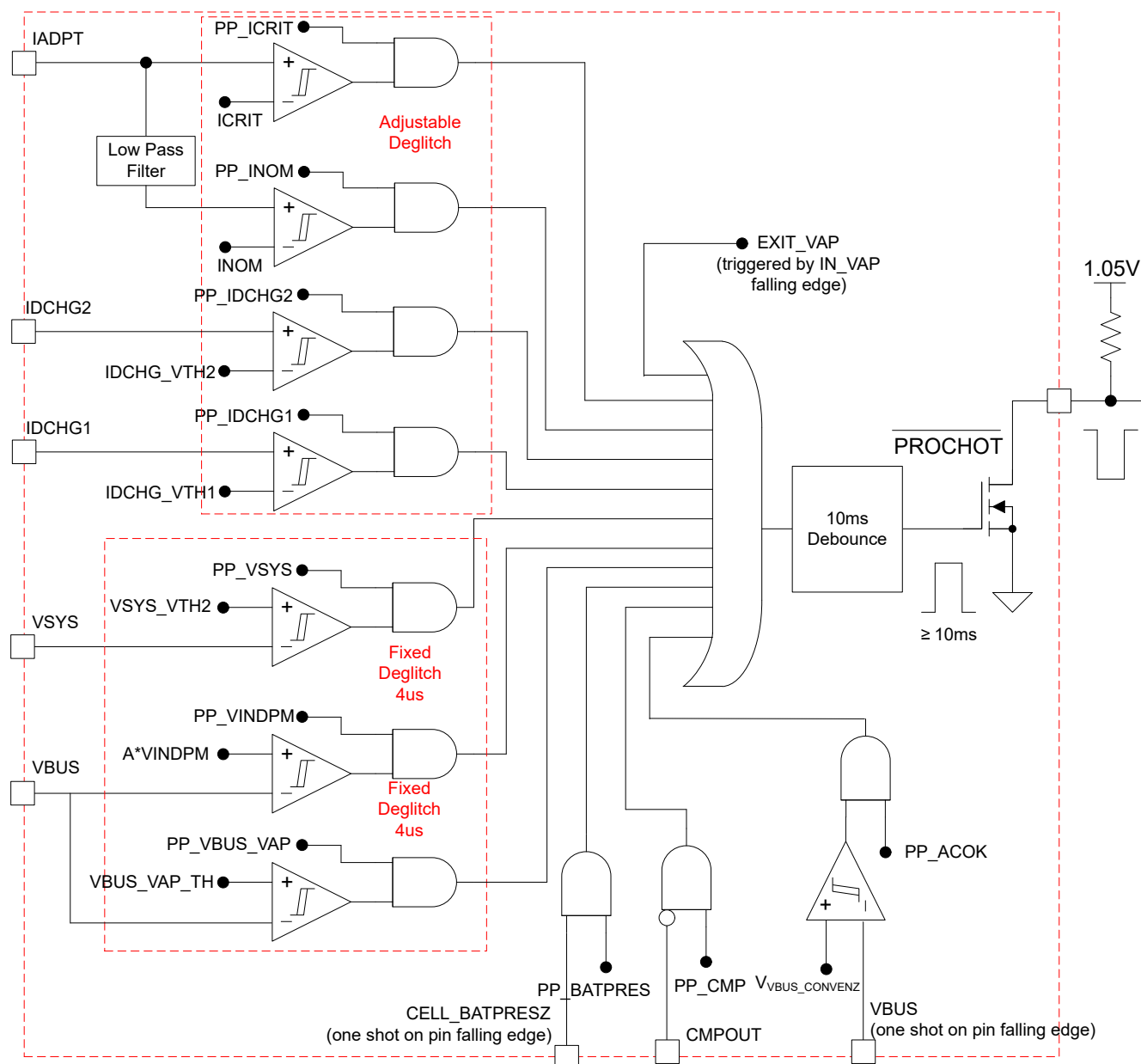
图 9-4. PROCHOT Profile
