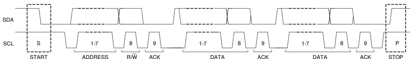
图 9-11. Complete Data Transfer
