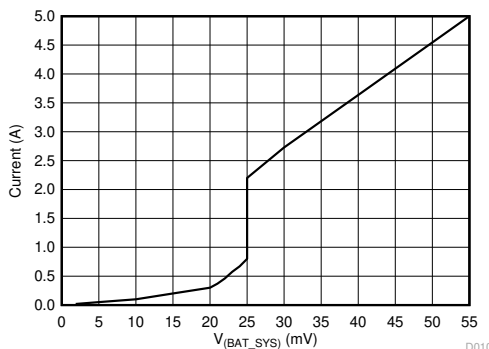
图 9-4. BATFET V-I Curve
