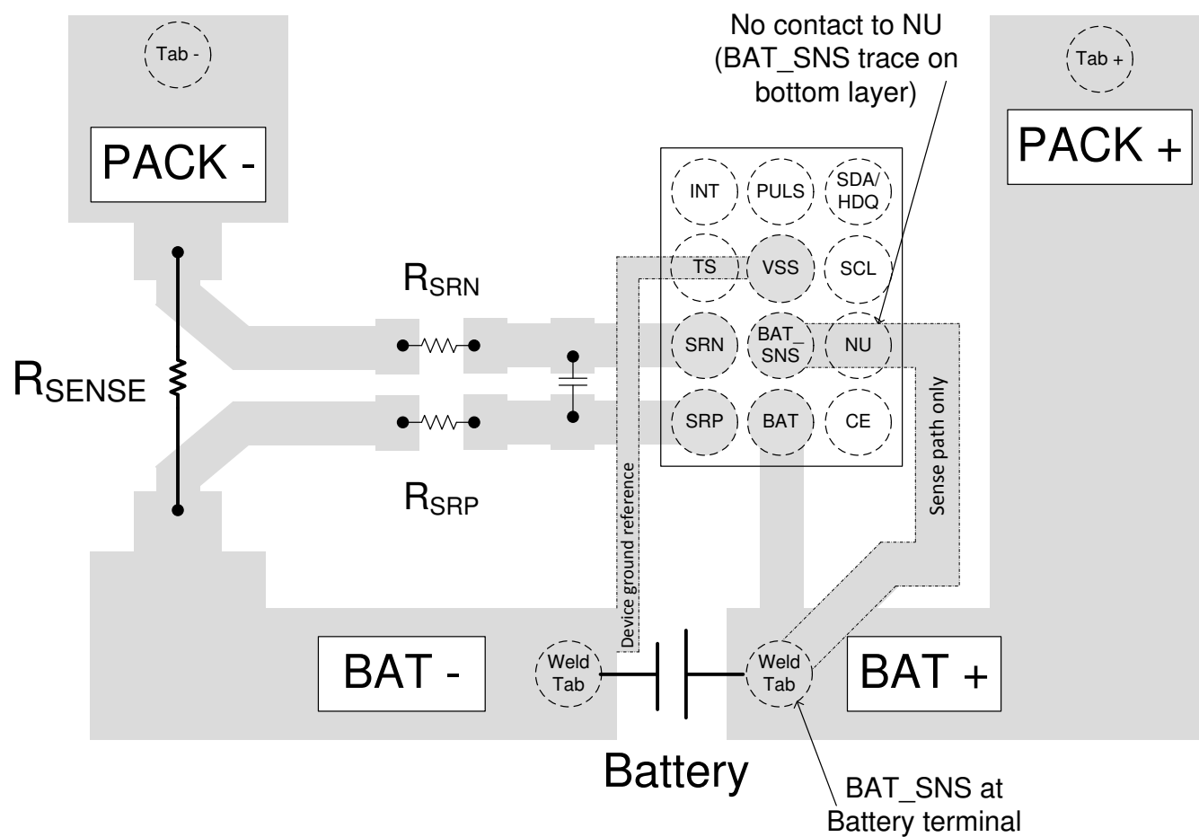
图 7-3. BQ27Z561 主要布线电路板布局布线
