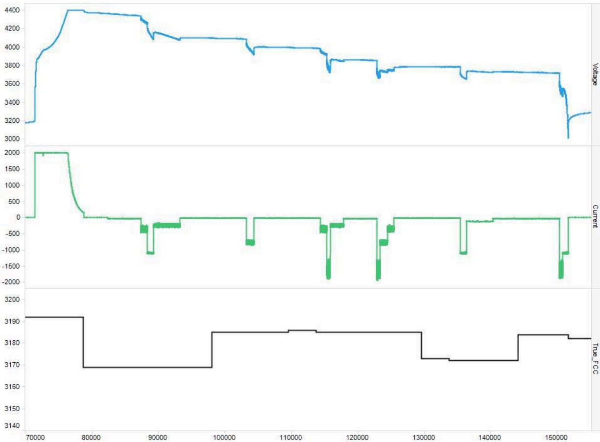
图 7-2. 充满电容量跟踪 ( X 轴为秒 )
