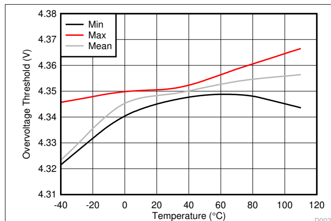
图 9-2. OVT vs Temperature
