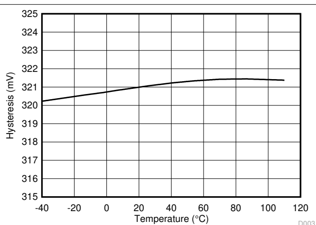
图 9-3. V_{HYS} vs Temperature
