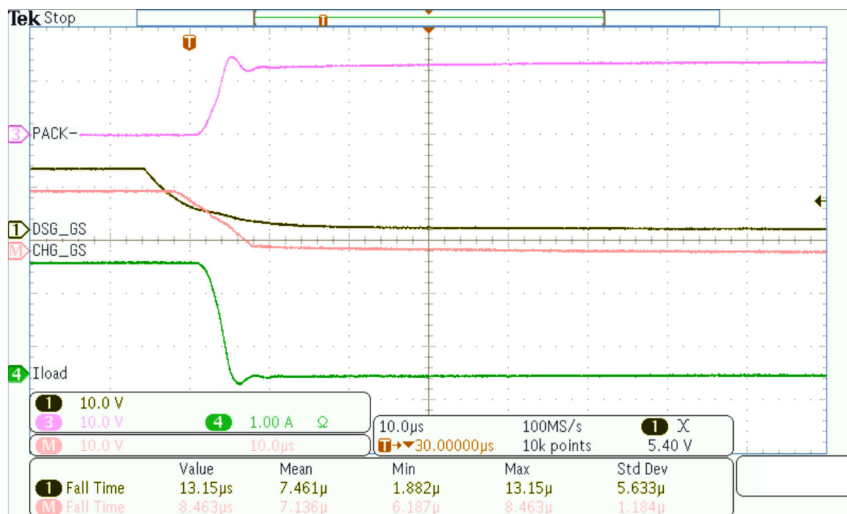
图 8-6. 中速 FET 关断，使用一个 1.35kΩ 串联栅极电阻器，并且 PACK+ 和 PACK- 之间具有 2A 负载。
