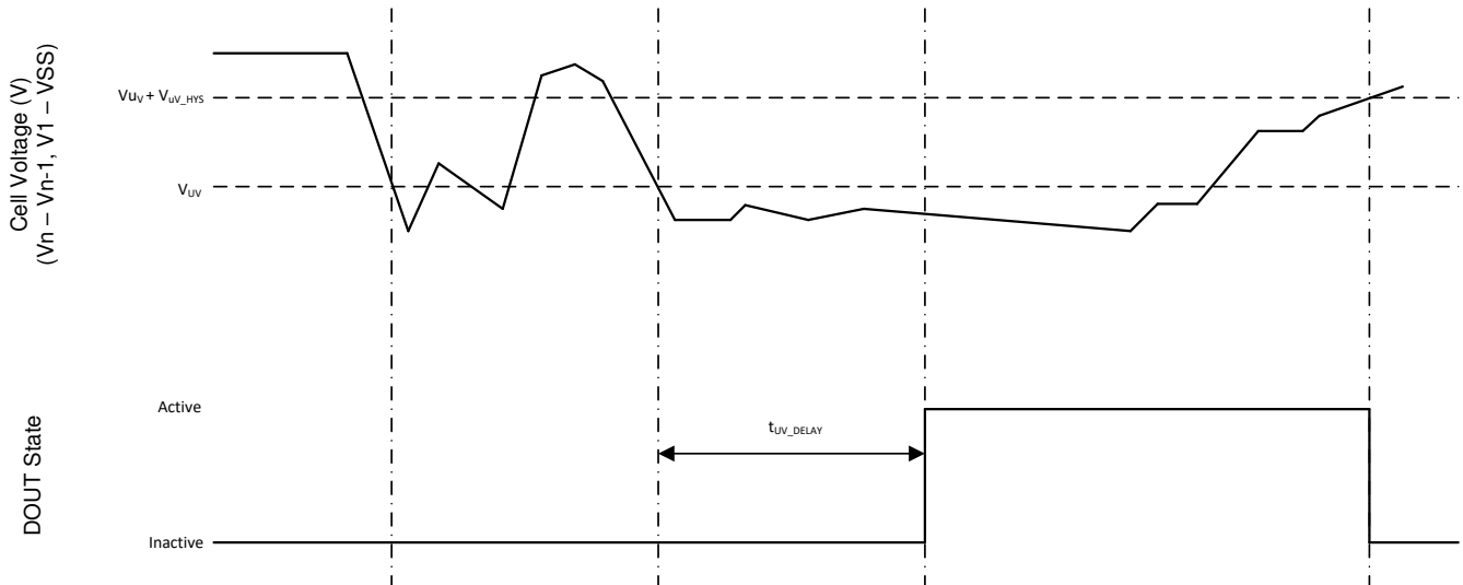
图 7-2. 欠压检测时序
