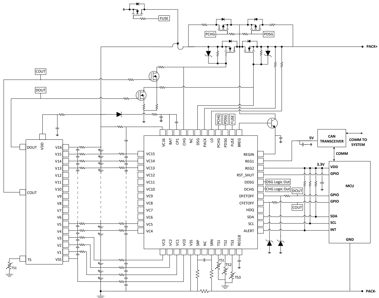
图 8-4. BQ77216 与 BQ76952
