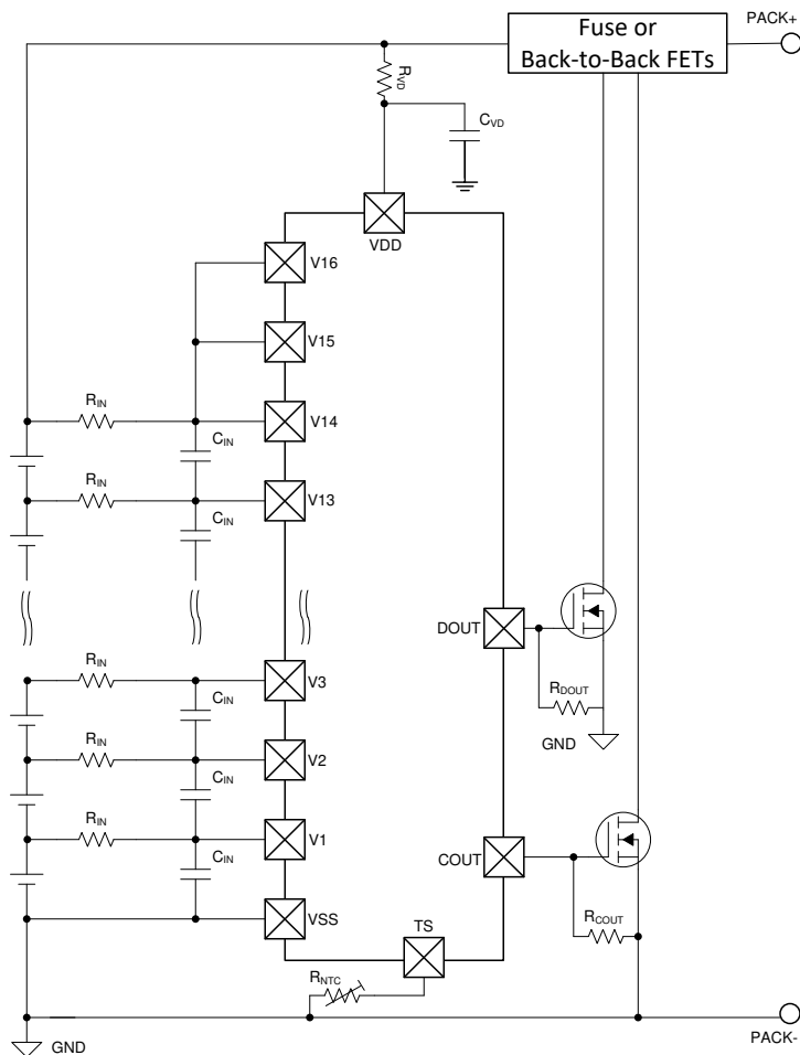
图 8-3. 具有高电平有效 6V 选项的 14 节串联电芯配置
