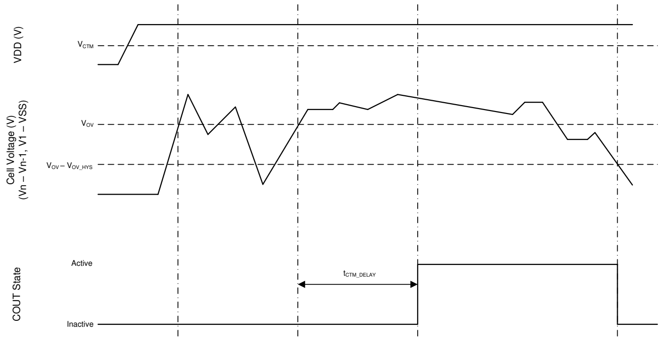
图 7-3. 客户测试模式的时序
