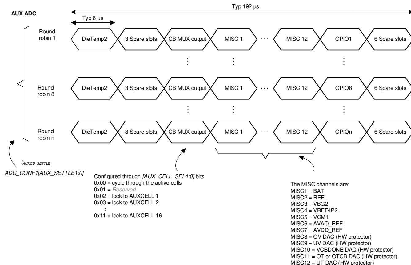
图 7-8. AUX ADC 轮询测量
