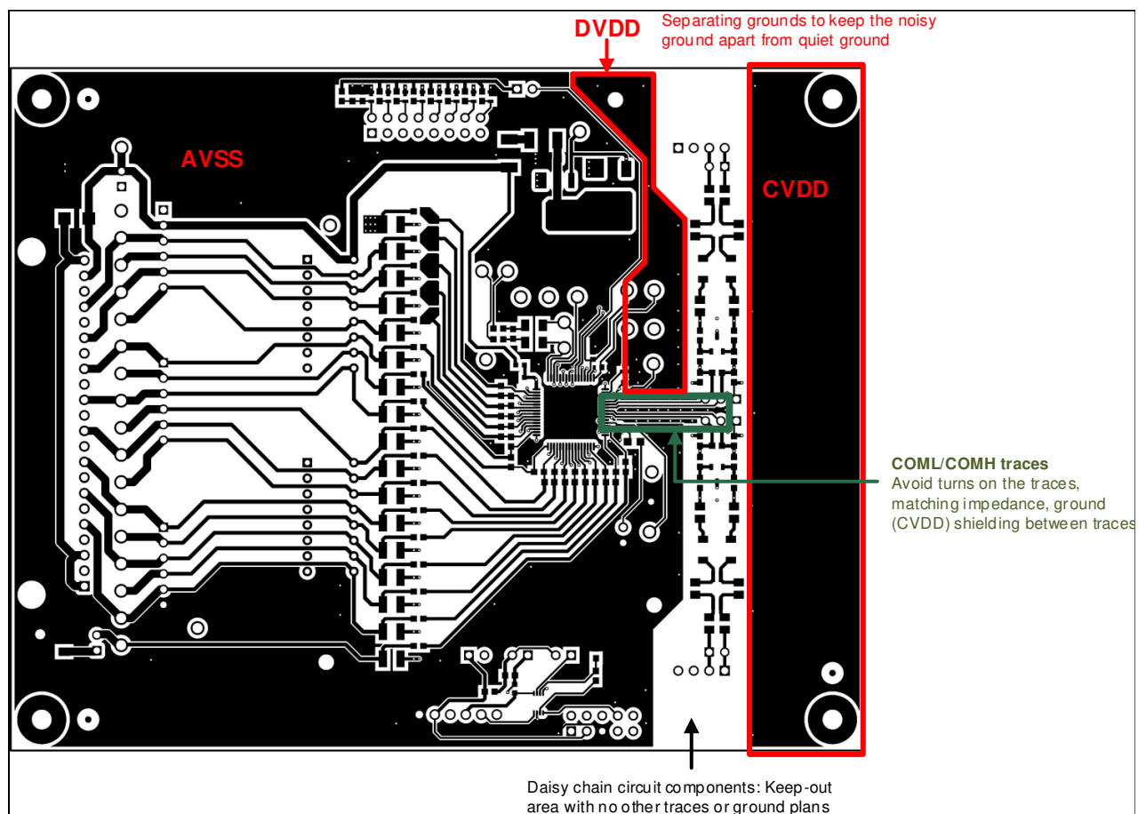
图 10-4. 顶端信号层
