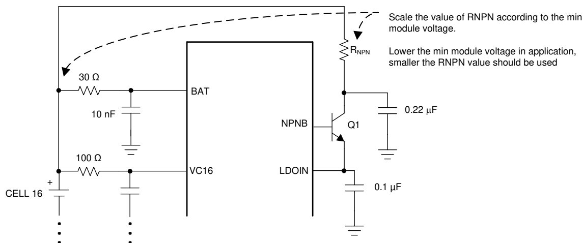
图 9-1. 器件供电路径
