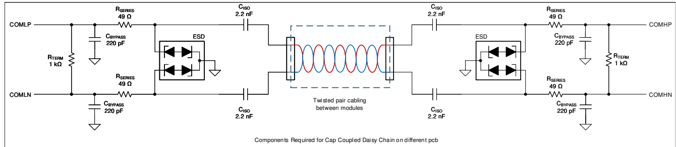
图 8-8. 不同 PCB 上的电容器隔离
