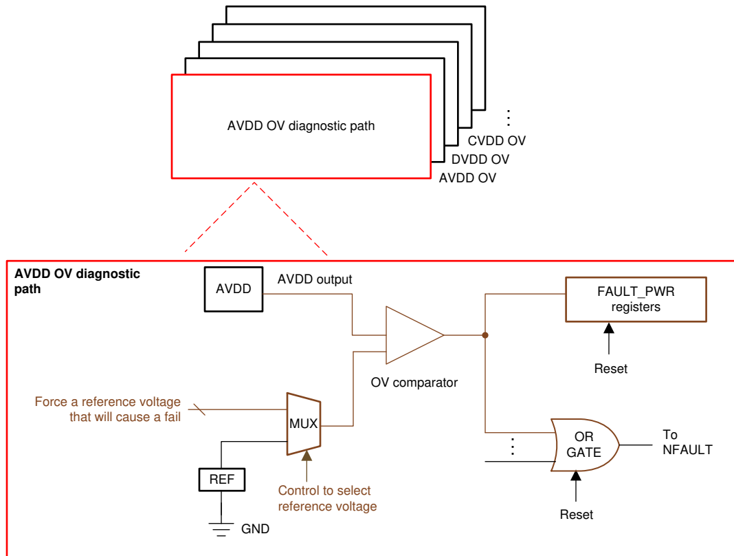
图 7-47. 电源 BIST
