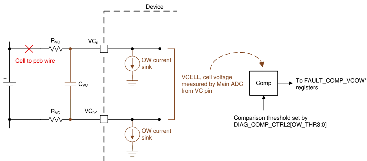
图 7-52. 开路检测
