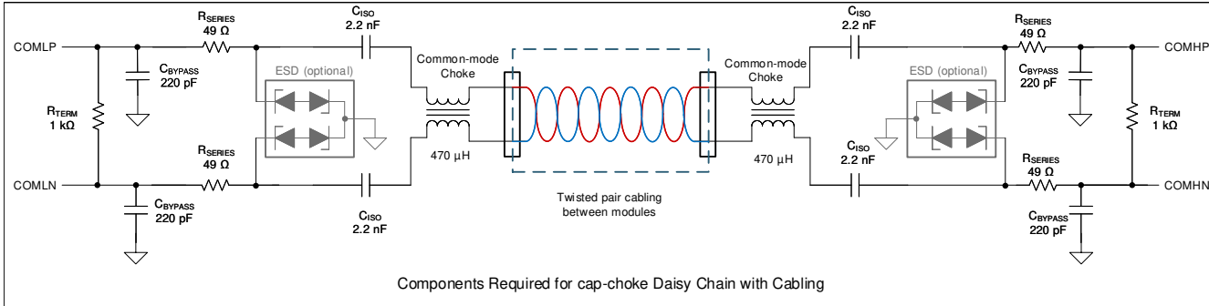
图 8-9. 电容器加扼流圈隔离
