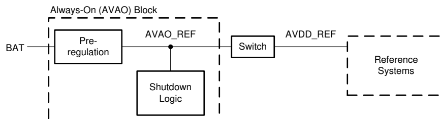
图 7-1. AVAO 块
