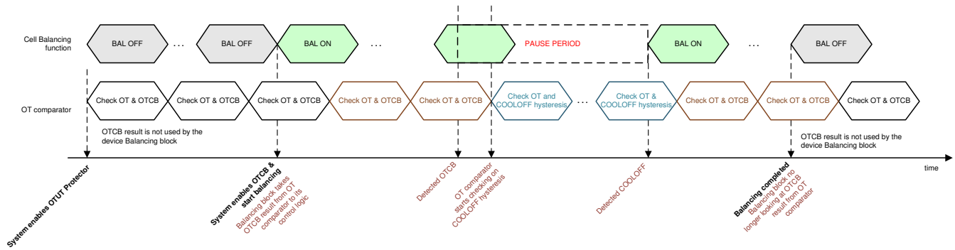
图 7-18. 通过 OTCB 检测暂停和恢复电芯均衡
