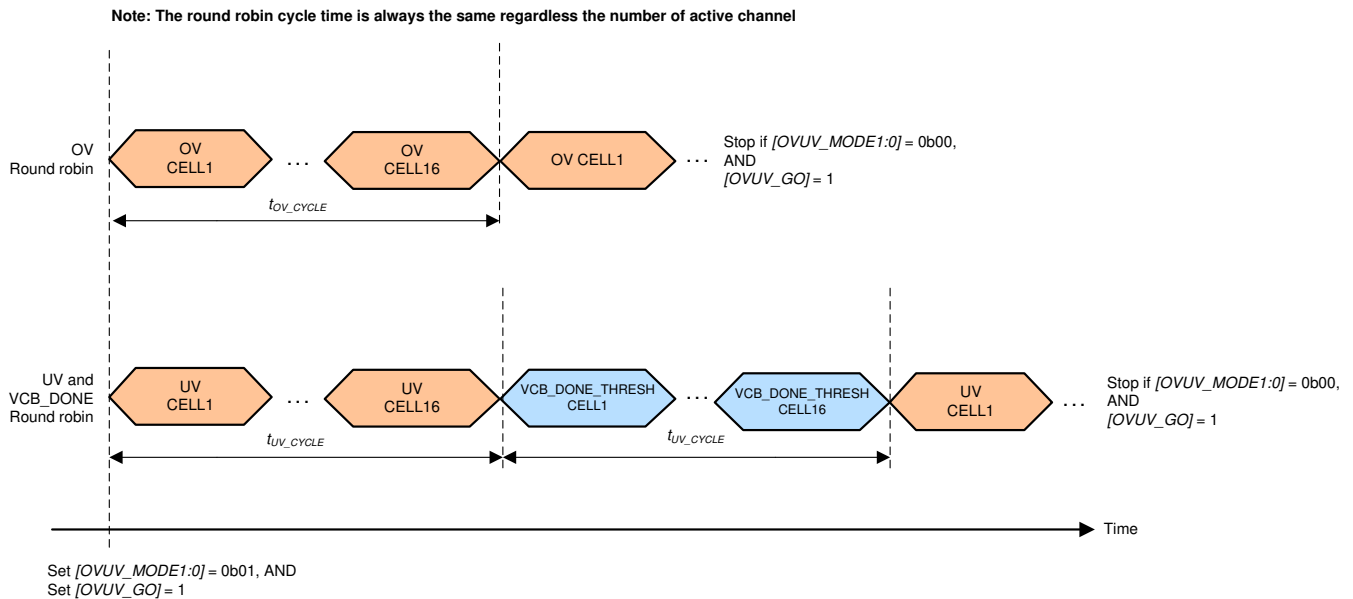
图 7-21. OV 和 UV 轮询模式
