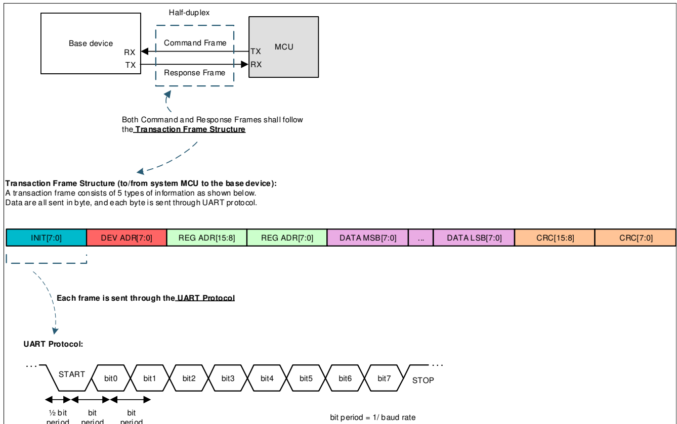
图 7-24. 与主机的 UART 通信
