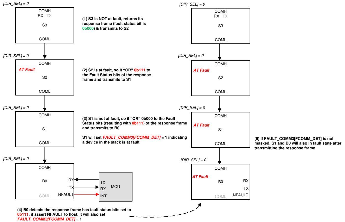
图 7-44. ACTIVE 模式下的传输故障状态 (响应单器件读取)
