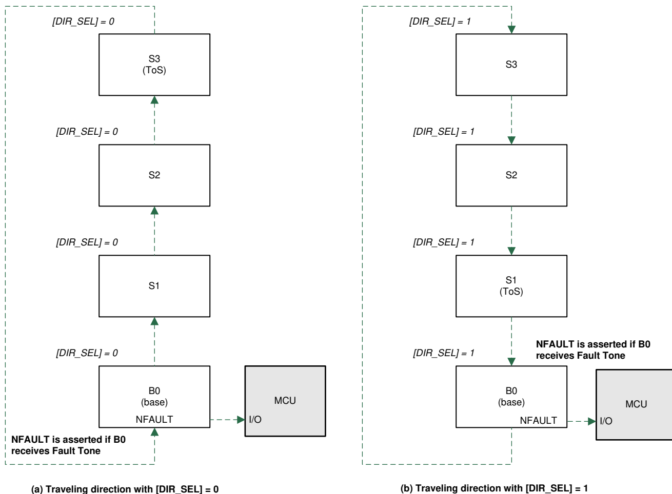
图 7-45. 检测信号或故障音调行进方向
