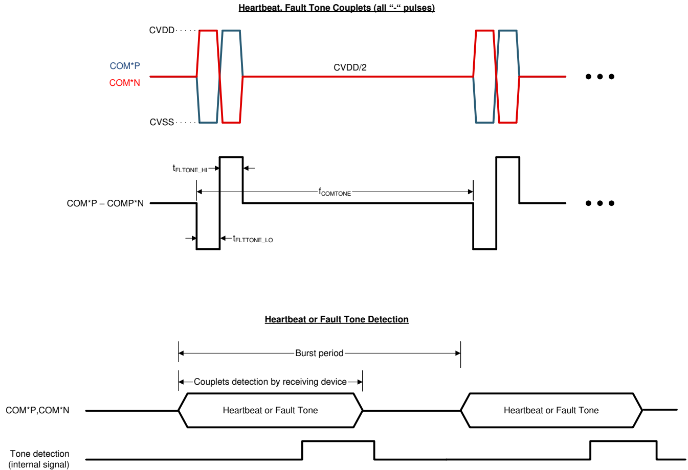
图 7-46. 检测信号和故障音调
