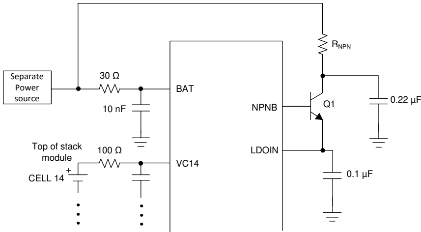
图 8-4. BAT 的单独电源
