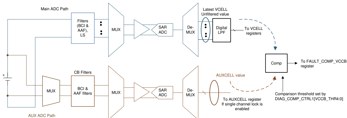
图 7-48. 电芯电压测量诊断
