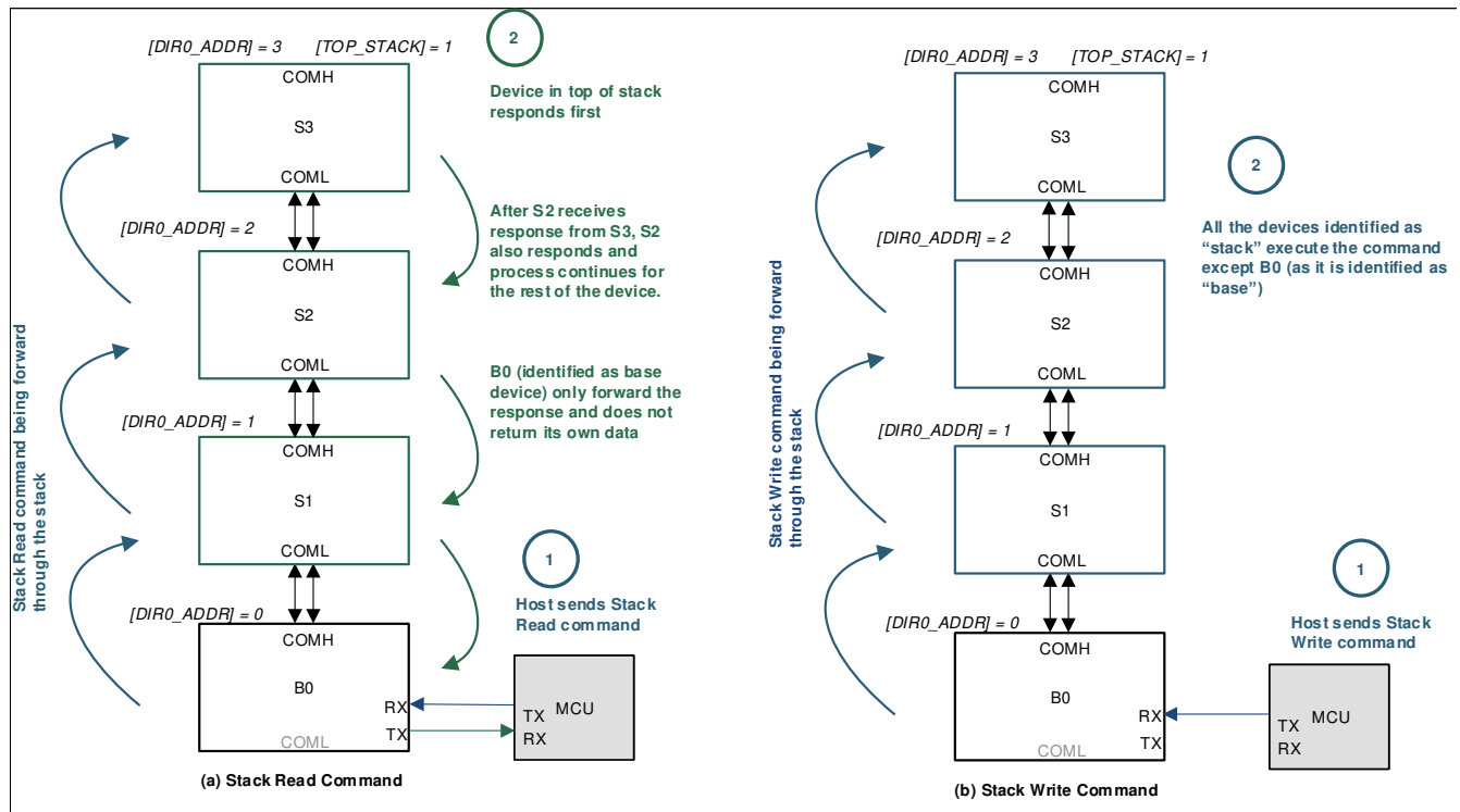
图 7-30. 堆栈读取/写入
