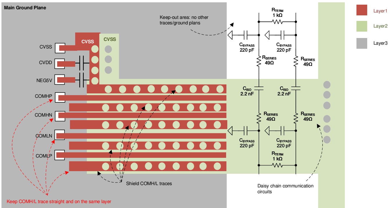
图 10-3. 菊花链布局注意事项
