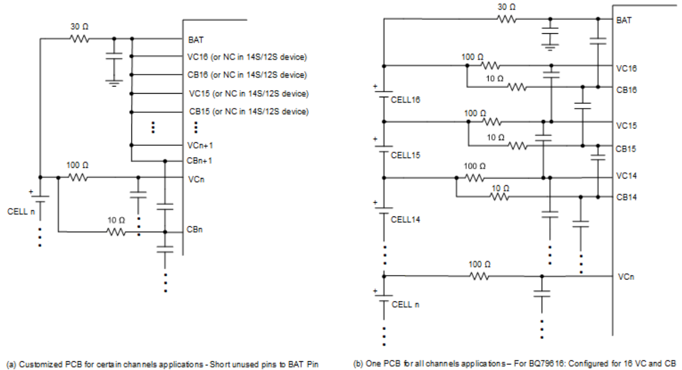
图 8-2. 未使用的 VC 和 CB 通道
