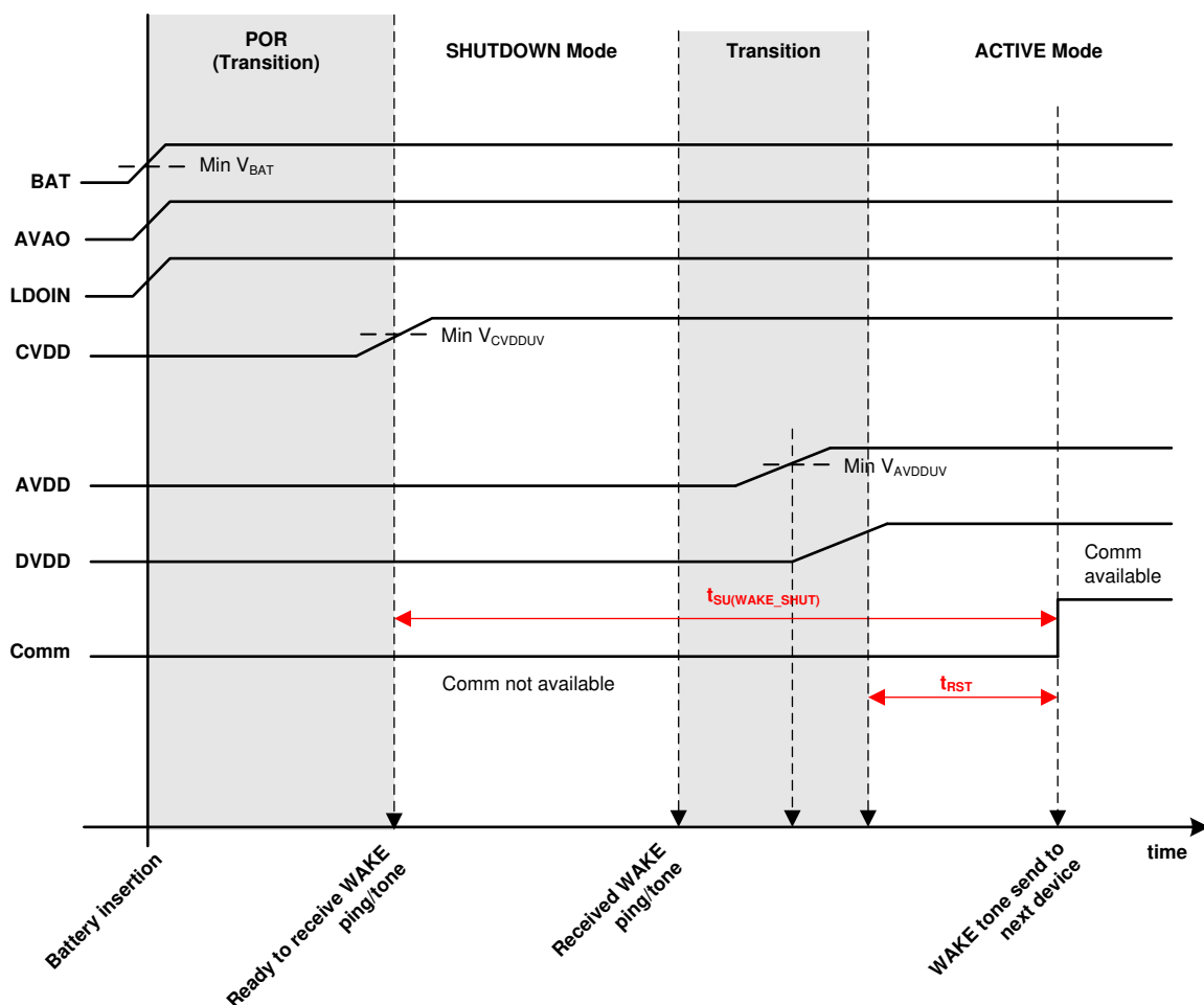
图 7-57. SHUTDOWN 至 ACTIVE 模式转换
