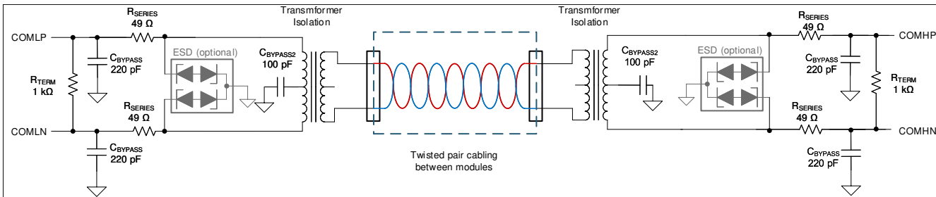
图 8-10. 变压器隔离
