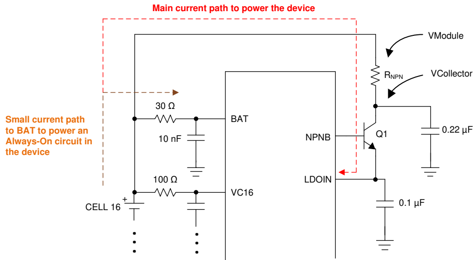
图 8-3. 功耗路径
