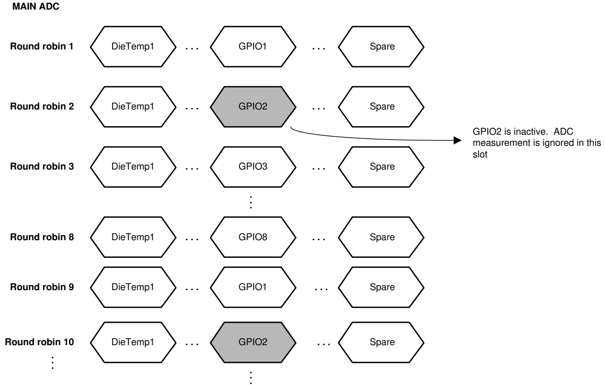
图 7-6. GPIO2 未配置用于 ADC 测量
