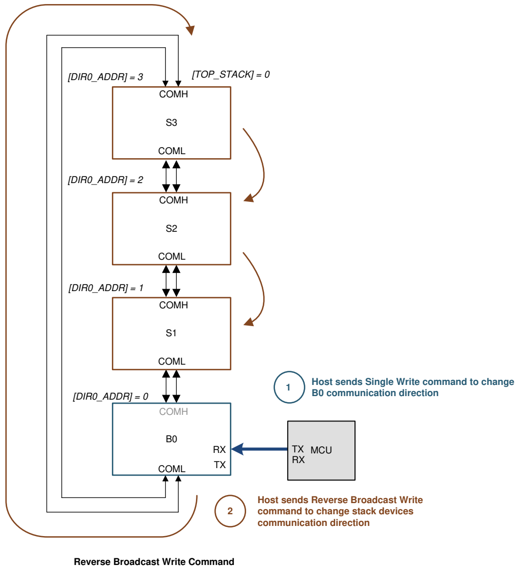
图 7-32. 广播写入反向
