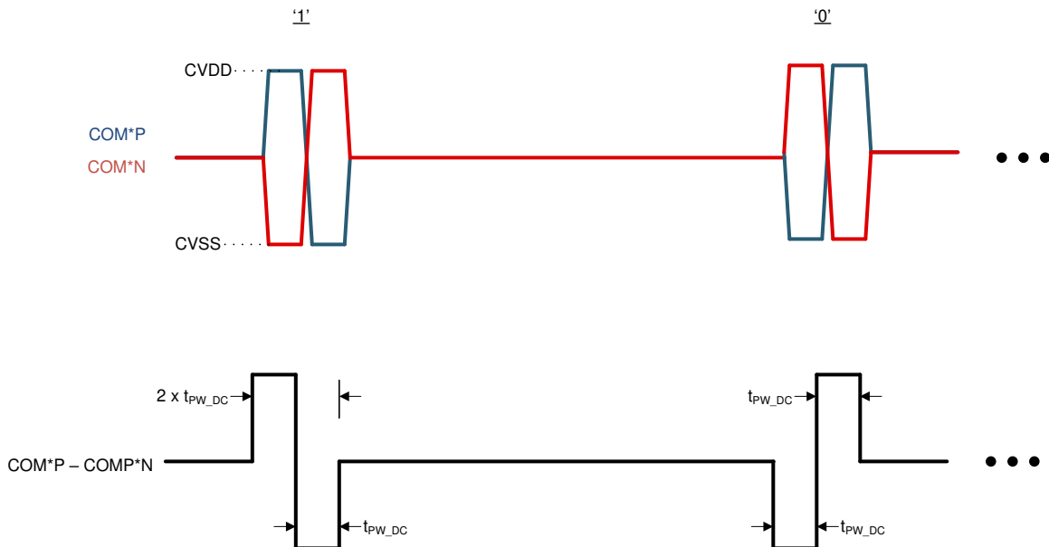
图 7-33. 菊花链位定义
