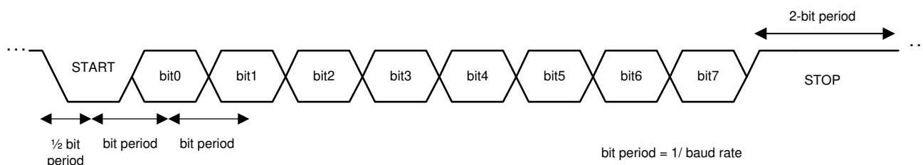
图 7-25. 具有两个 STOP 位的 UART 响应帧
