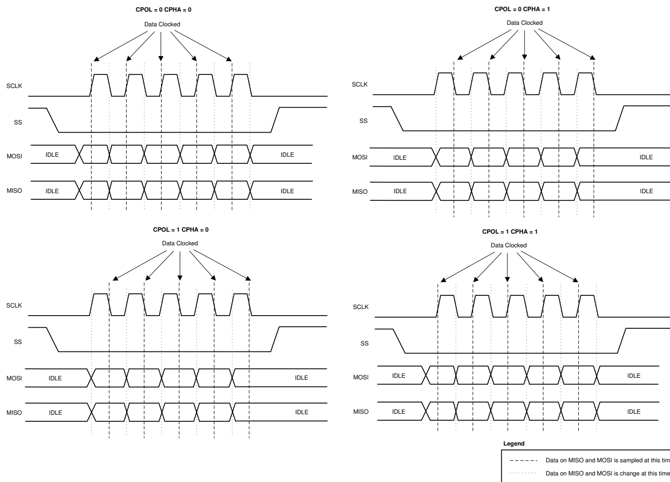
图 7-41. SPI 主器件 CPOL 和 CPHA
