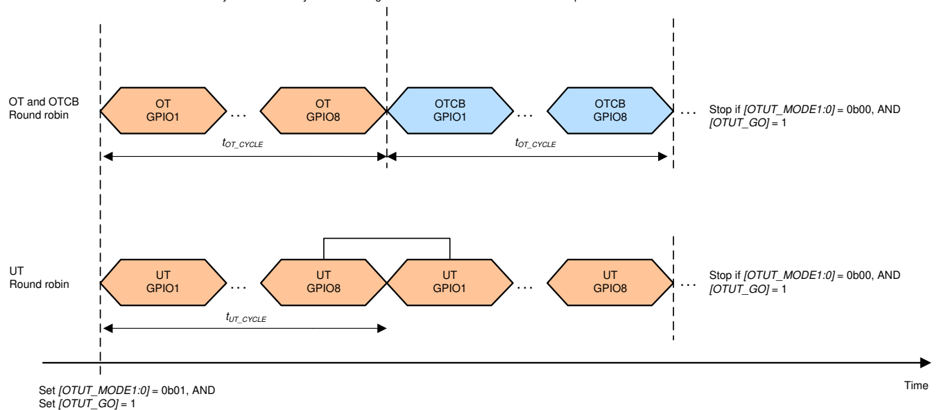
图 7-23. OT 和 UT 轮询模式
