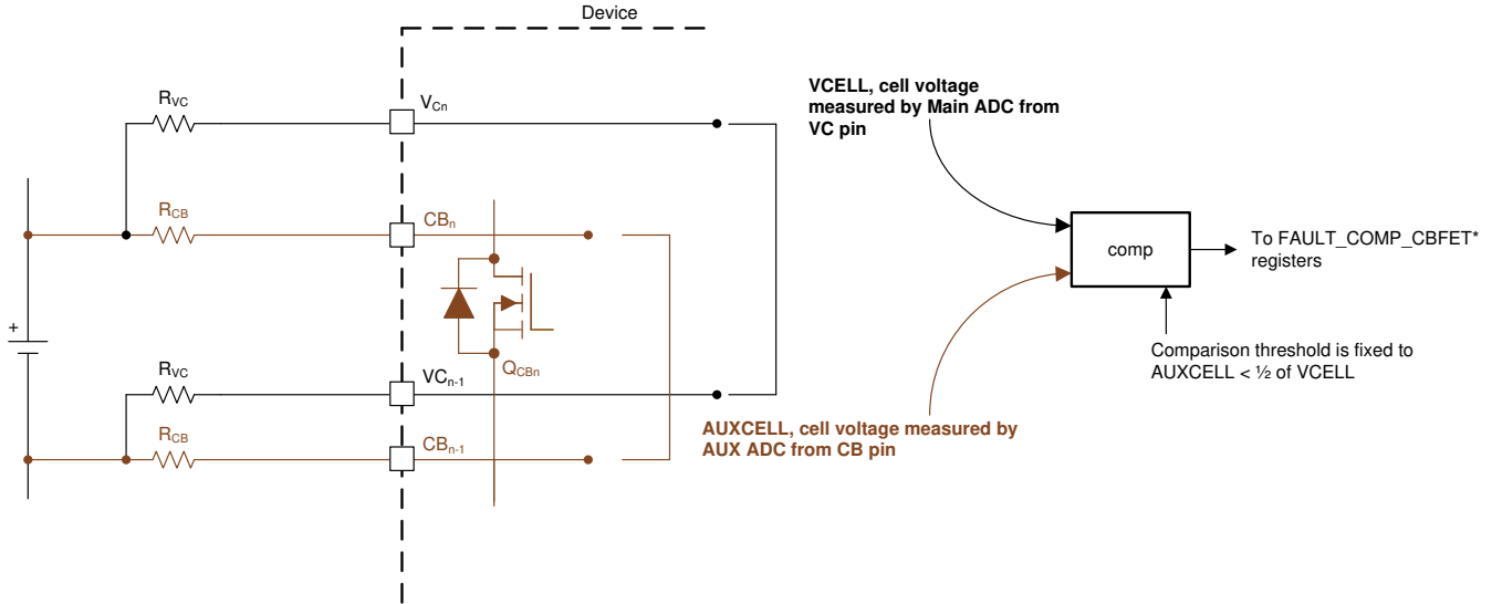
图 7-51. 电芯均衡 FET 诊断
