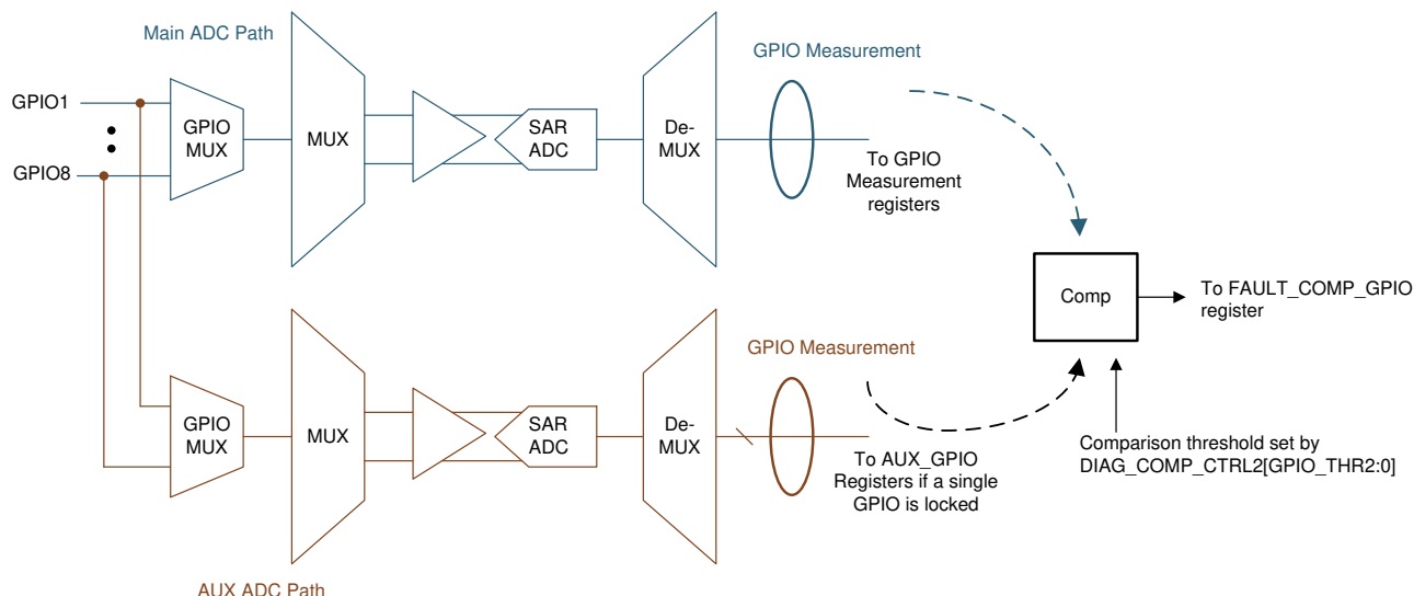
图 7-50. 热敏电阻温度 (GPIO) 测量诊断
