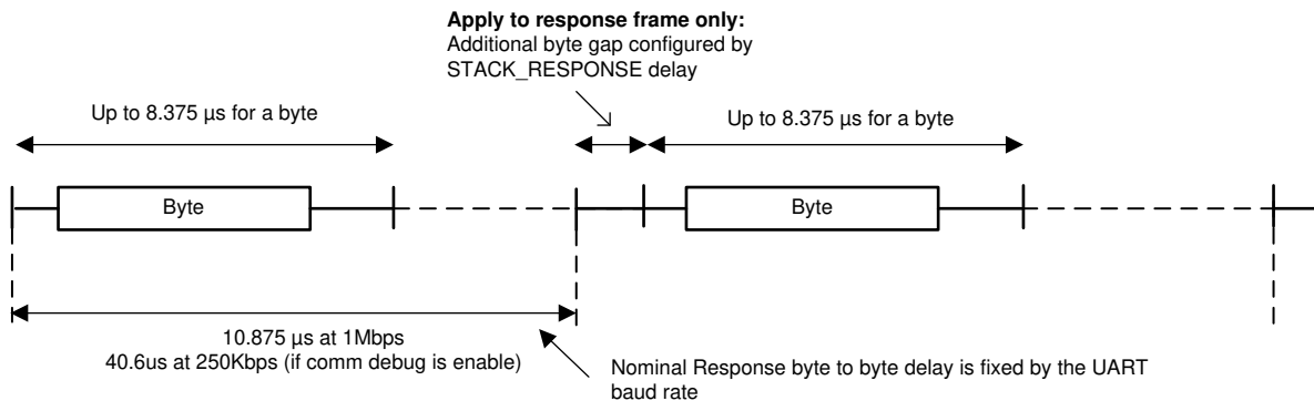
图 7-35. 菊花链字节传输
