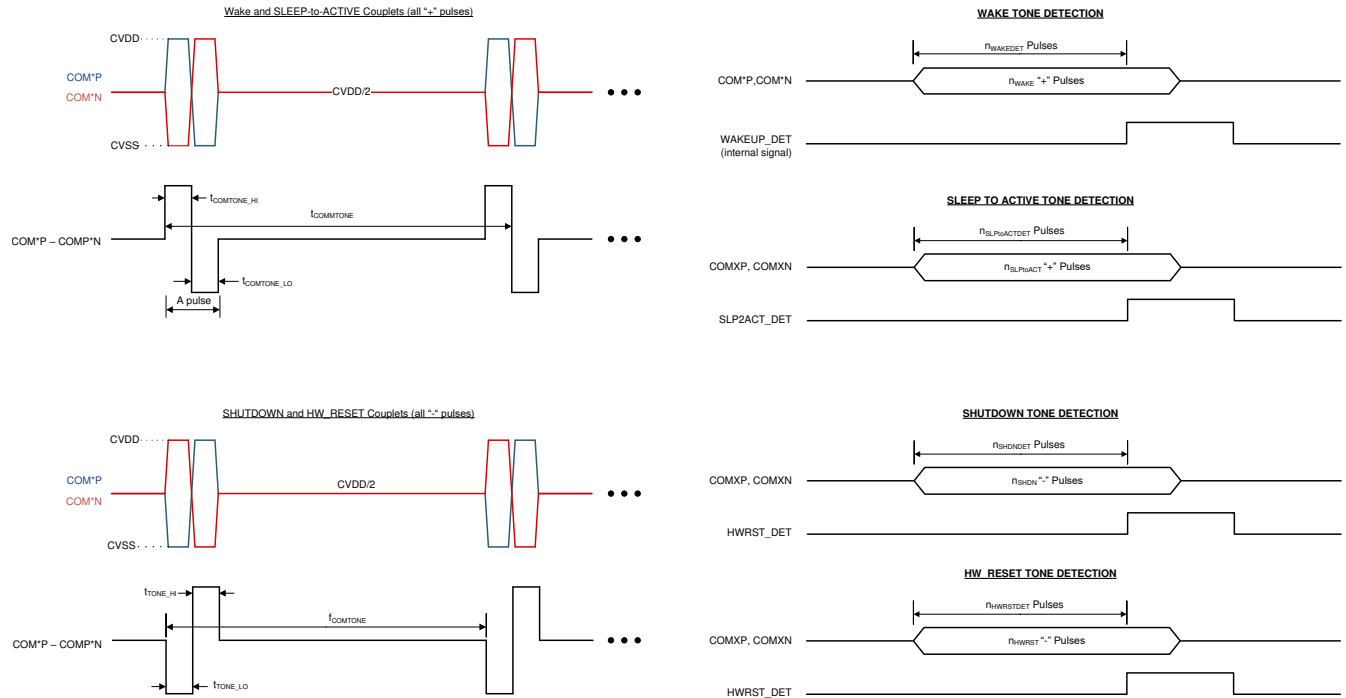
图 7-60. 通信音调
