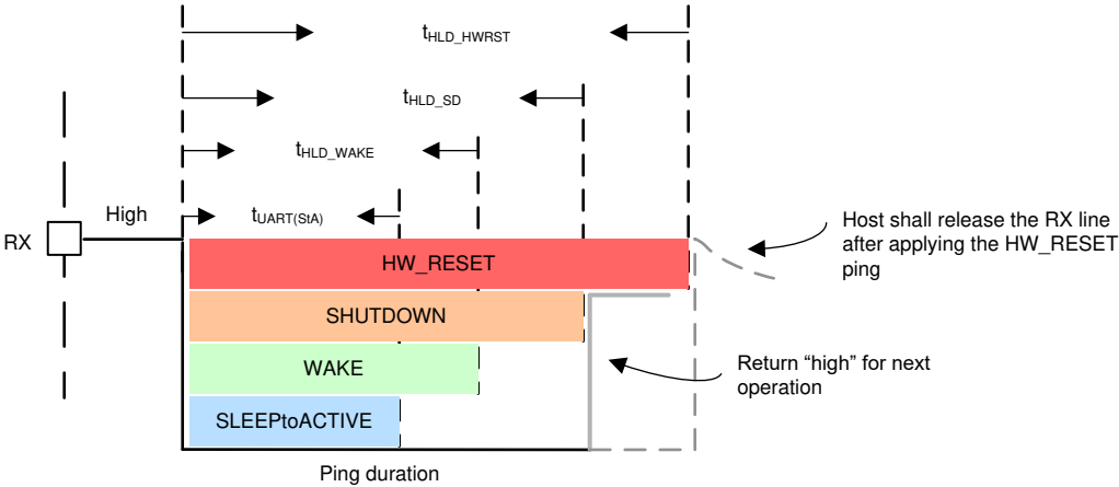
图 7-59. 通信 ping
