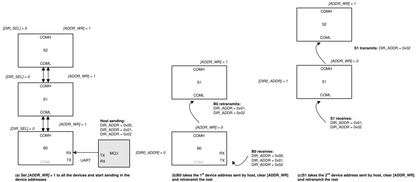
图 7-37. 自动寻址
