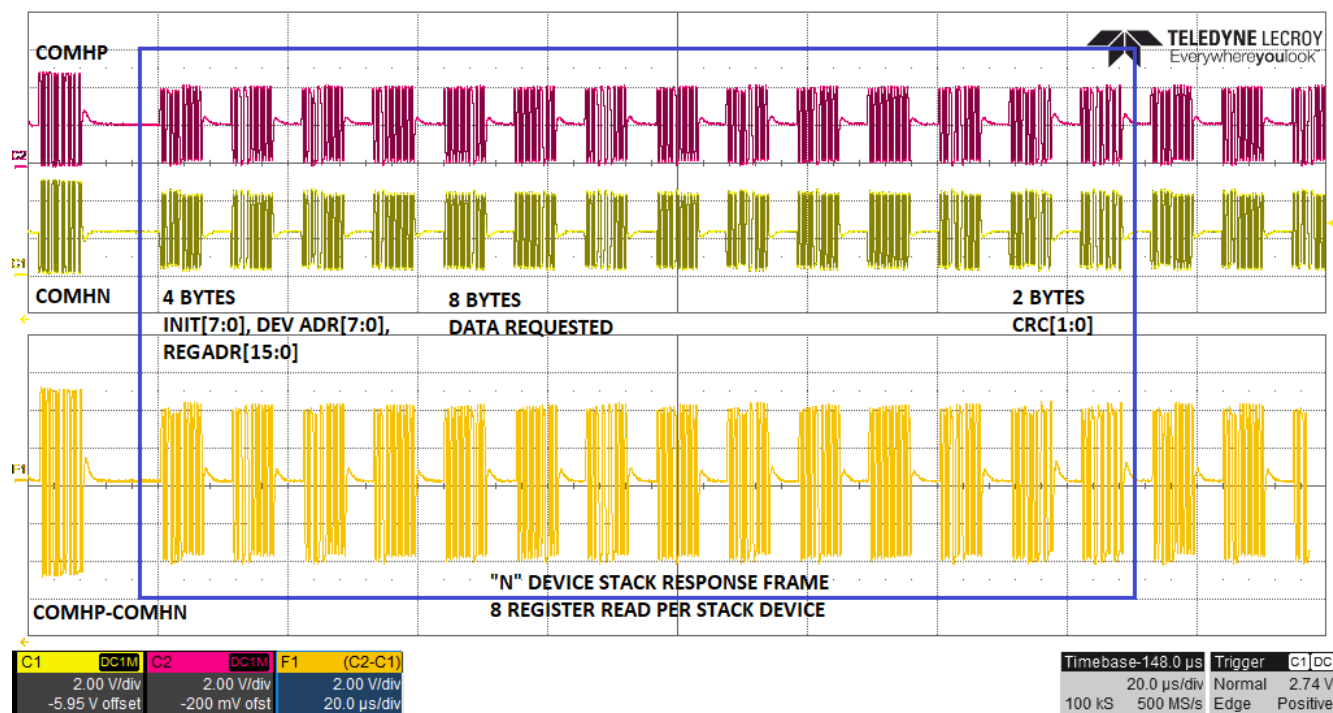
图 8-11. 从堆栈器件读取 8 个寄存器的响应帧
