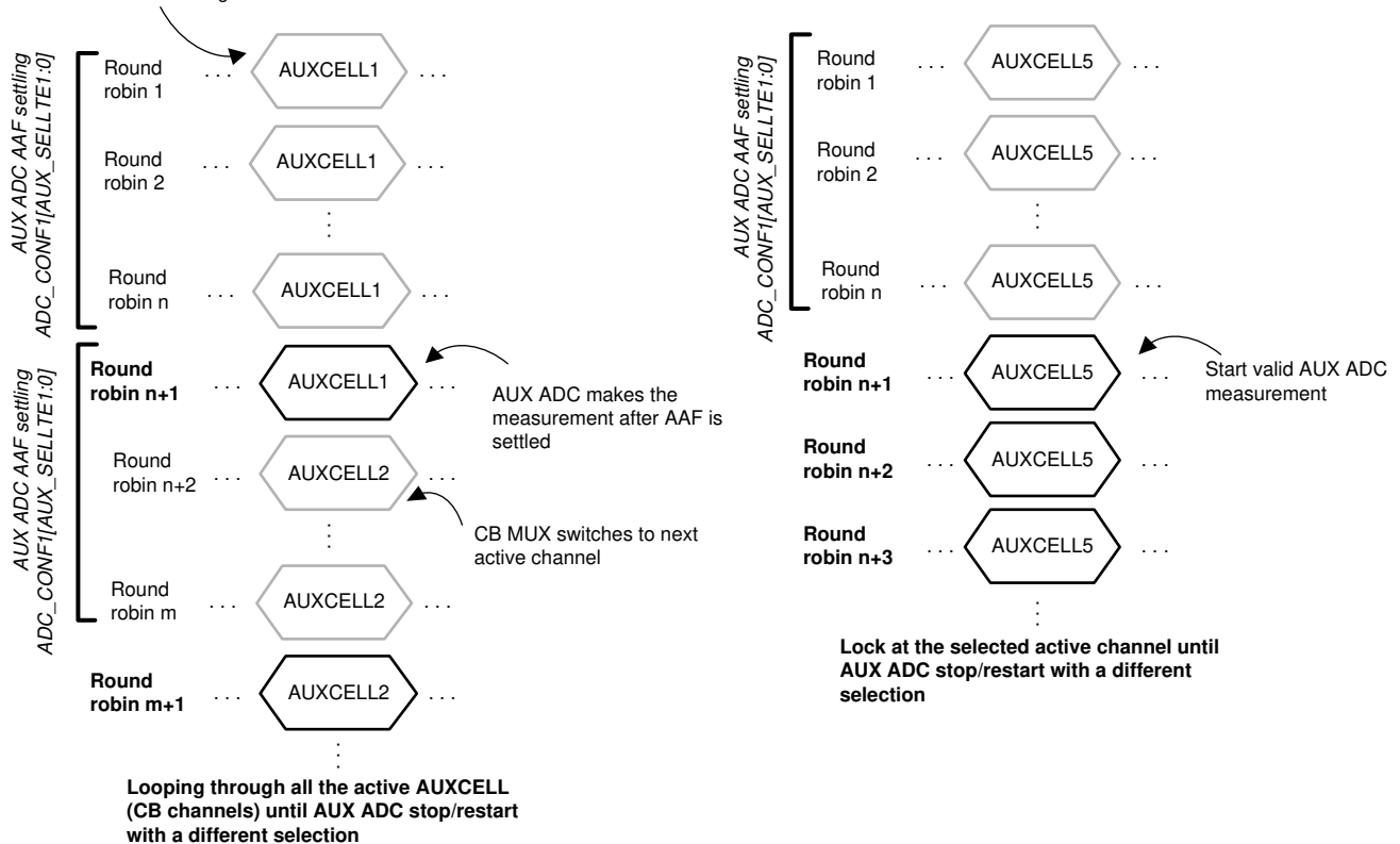
图 7-9. 具有不同 [AUX_CELL_SEL4:0] 设置的 CB 多路复用器输出时隙
