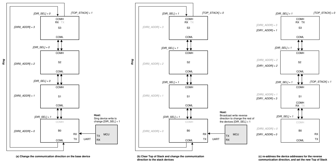
图 7-38. 更改菊花链中的通信方向的示例
