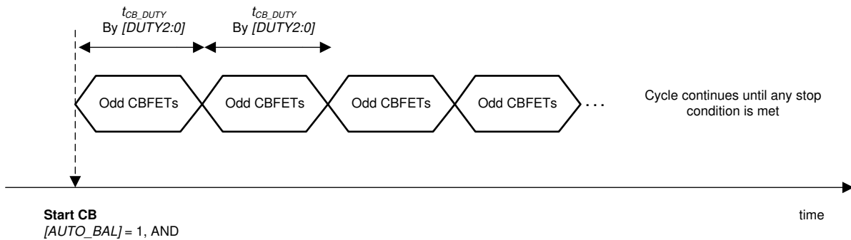
图 7-16. 自动均衡控制，示例 2
