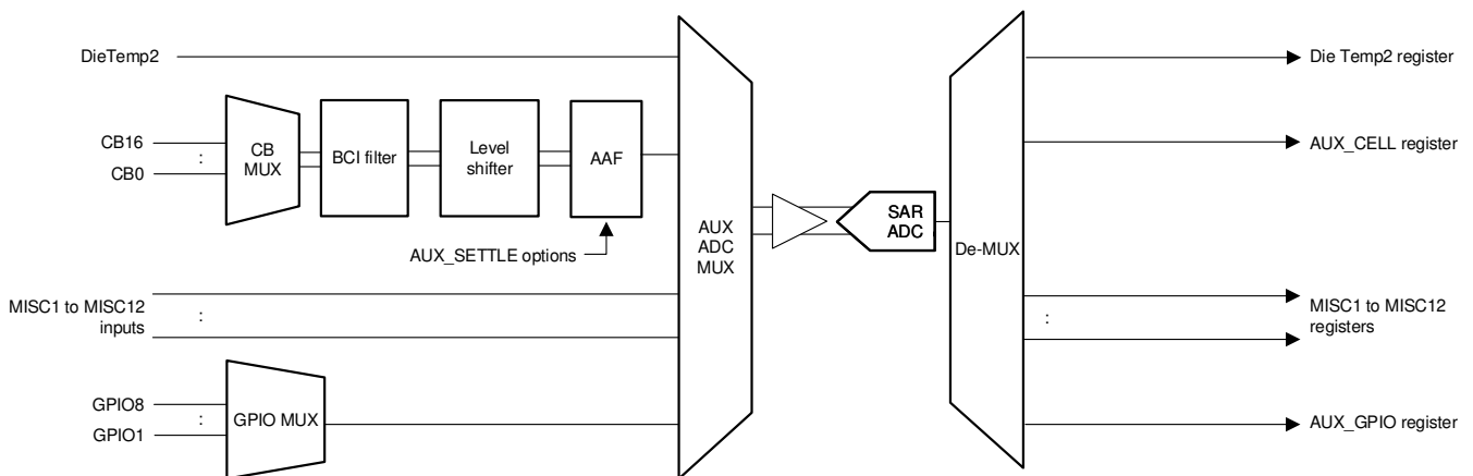
图 7-7. AUX ADC 测量路径
