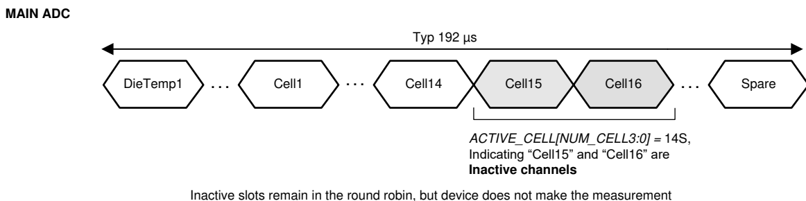
图 7-4. 6S 至 16S 具有相同的轮询时序
