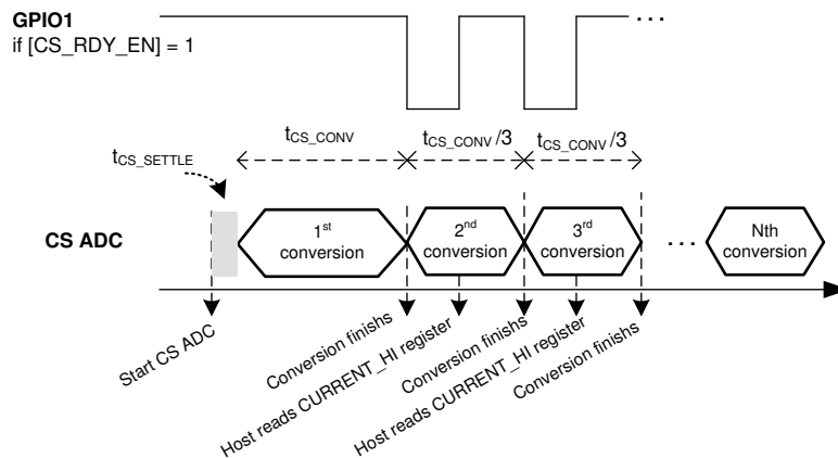
图 7-13. CS ADC 测量
