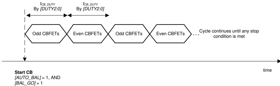
图 7-15. 自动均衡控制，示例 1
