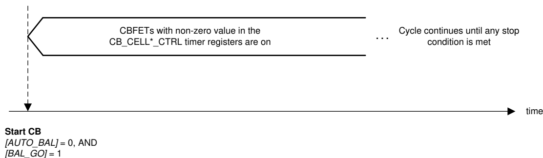
图 7-17. 手动均衡控制
