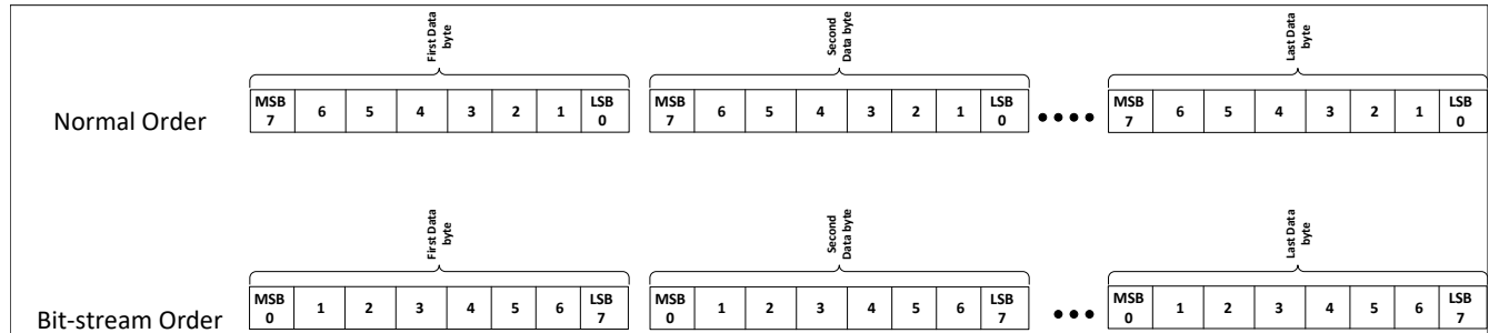
图 7-28. 位流顺序说明
