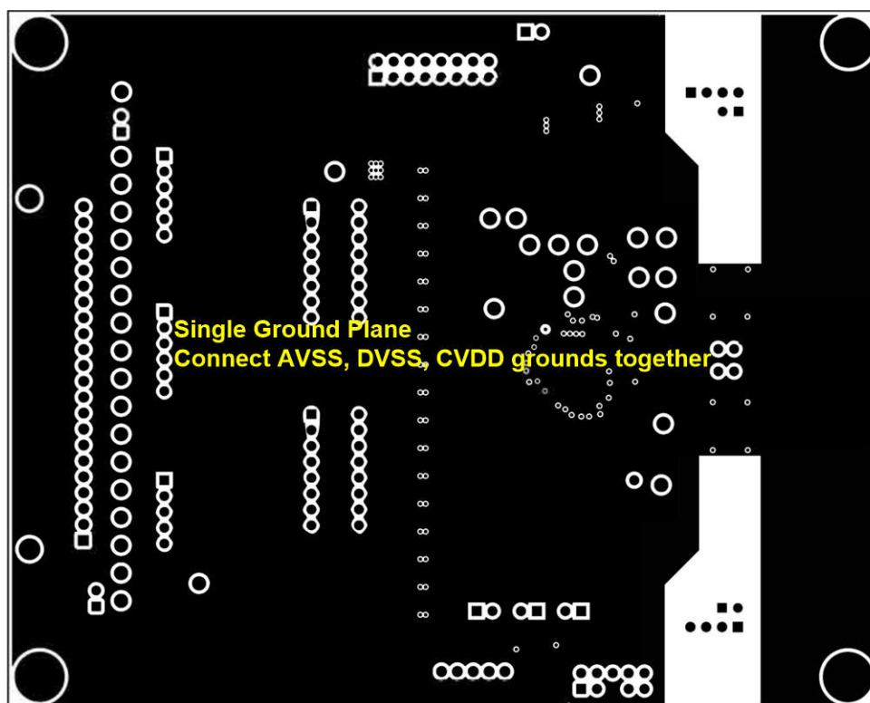
图 10-6. 具有单个接地平面的第三层
