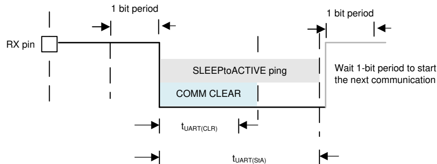
图 7-27. UART COMM CLEAR
