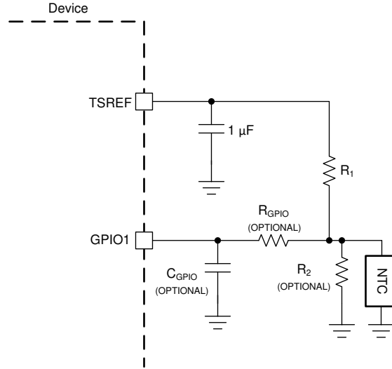
图 8-5. NTC 连接
