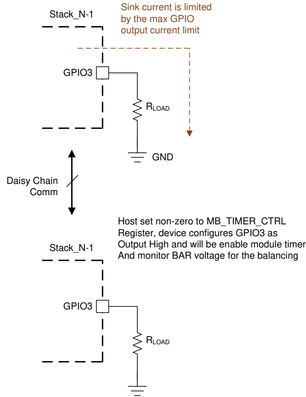
图 7-19. 模块均衡
