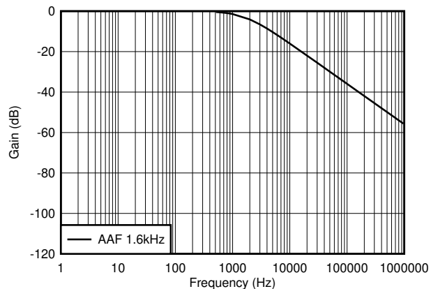
图 6-5. 主 ADC 滤波器
