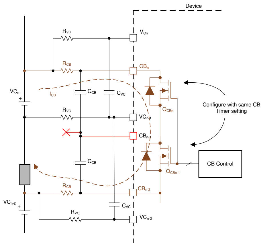
图 7-54. 通过连接到单独 VC 通道的汇流条进行电芯均衡
