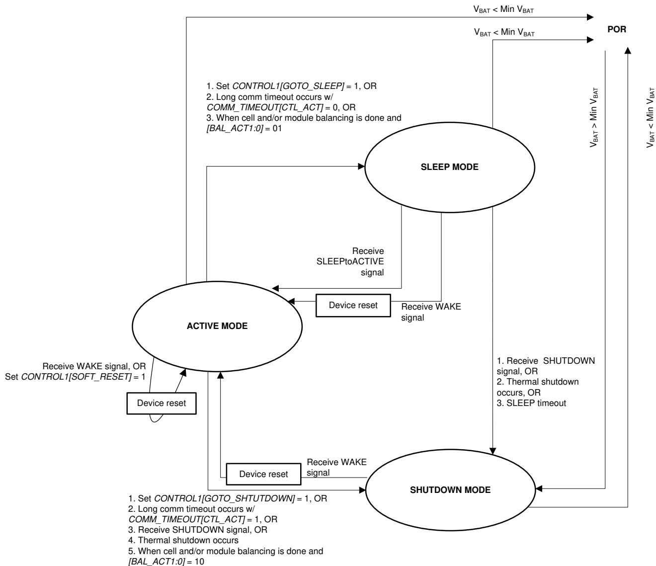
图 7-56. 功耗状态图
