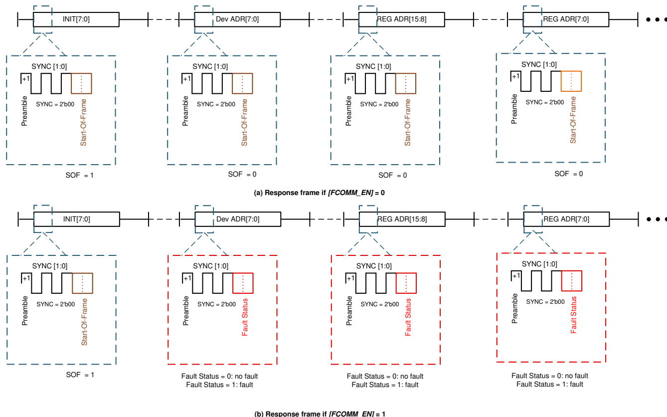
图 7-43. 在通信响应帧中嵌入故障状态
