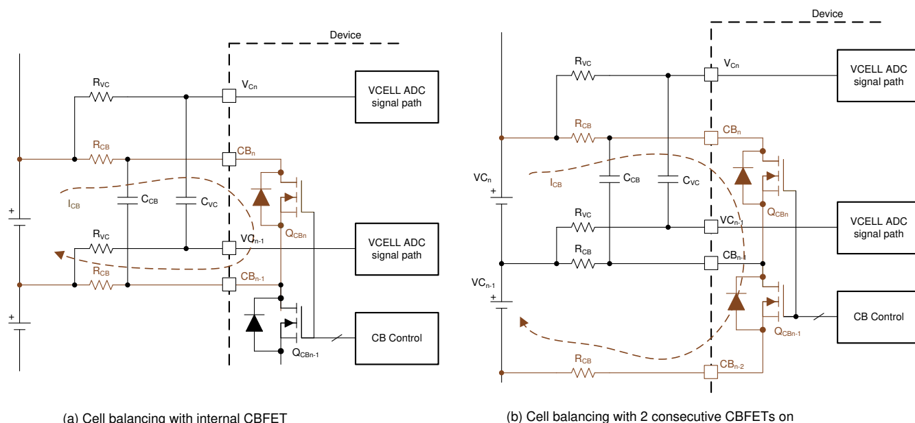
图 7-14. 内部电芯均衡和均衡电流的流动
