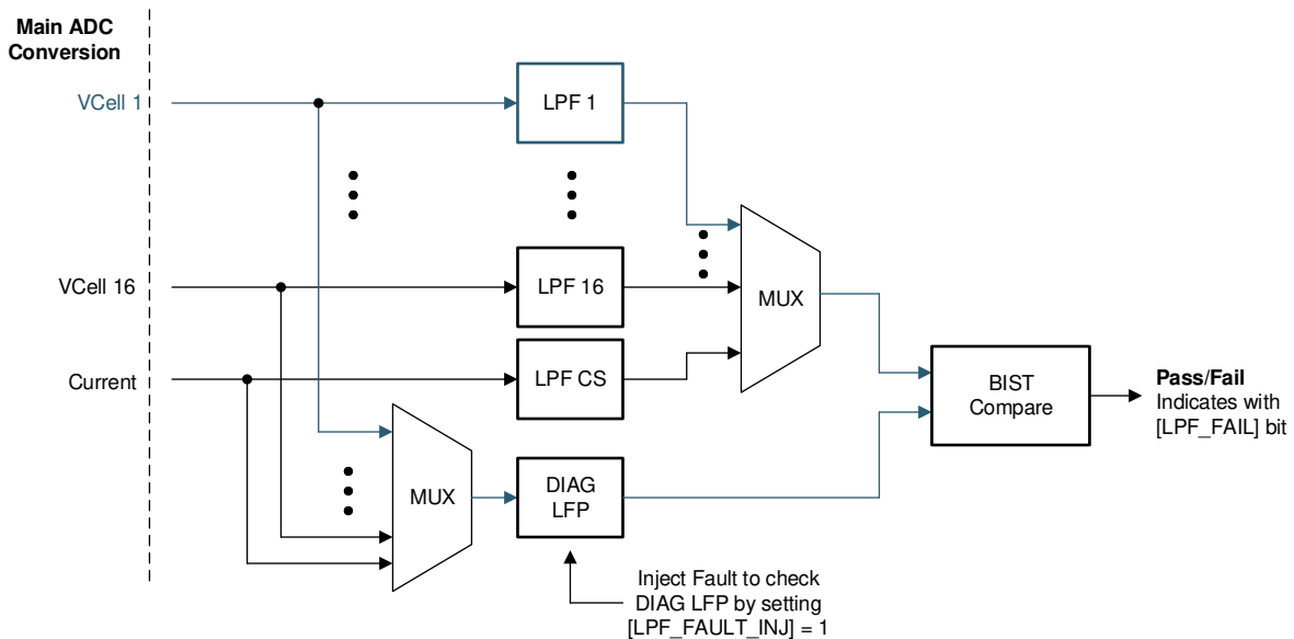
图 7-49. 后 ADC LPF 诊断 (蓝色路径是检查 LPF1 的示例)
