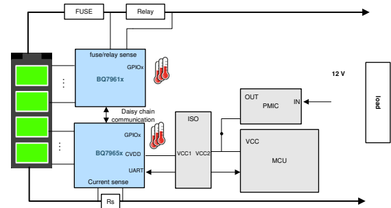
简化版系统图
