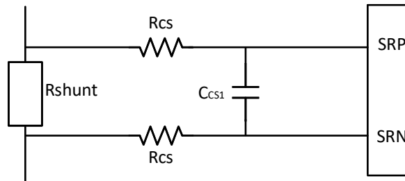
图 8-6. 电流检测输入连接
