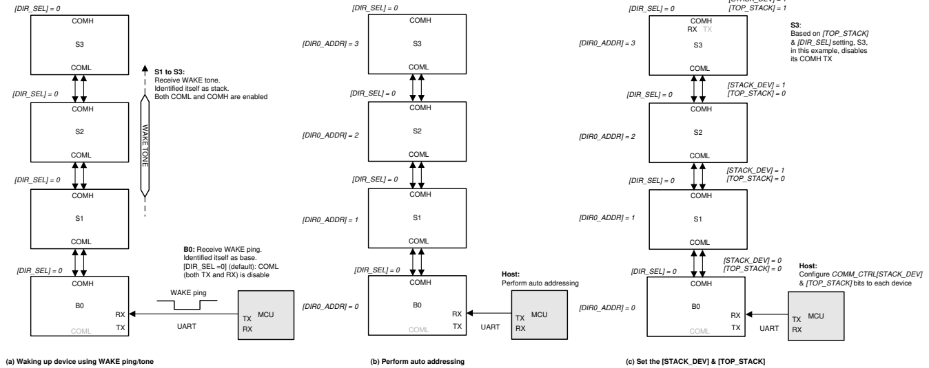
图 7-36. 配置器件进行通信
