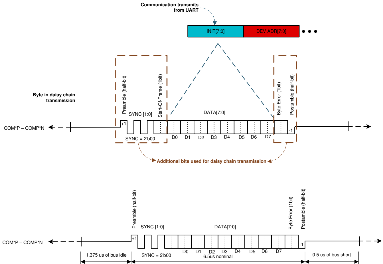
图 7-34. 菊花链字节定义
