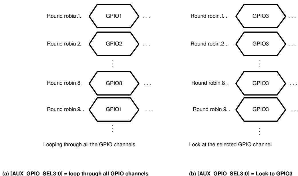
图 7-10. 具有不同 [AUX_GPIO_SEL3:0] 设置的 GPIO 时隙
