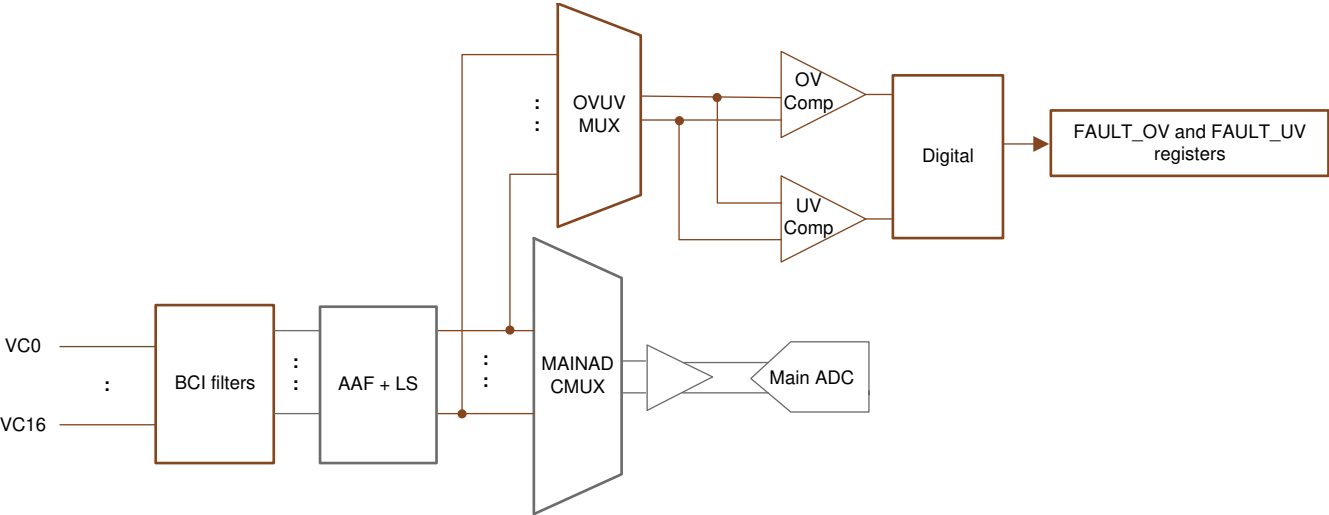
图 7-20. OV 和 UV 保护器
