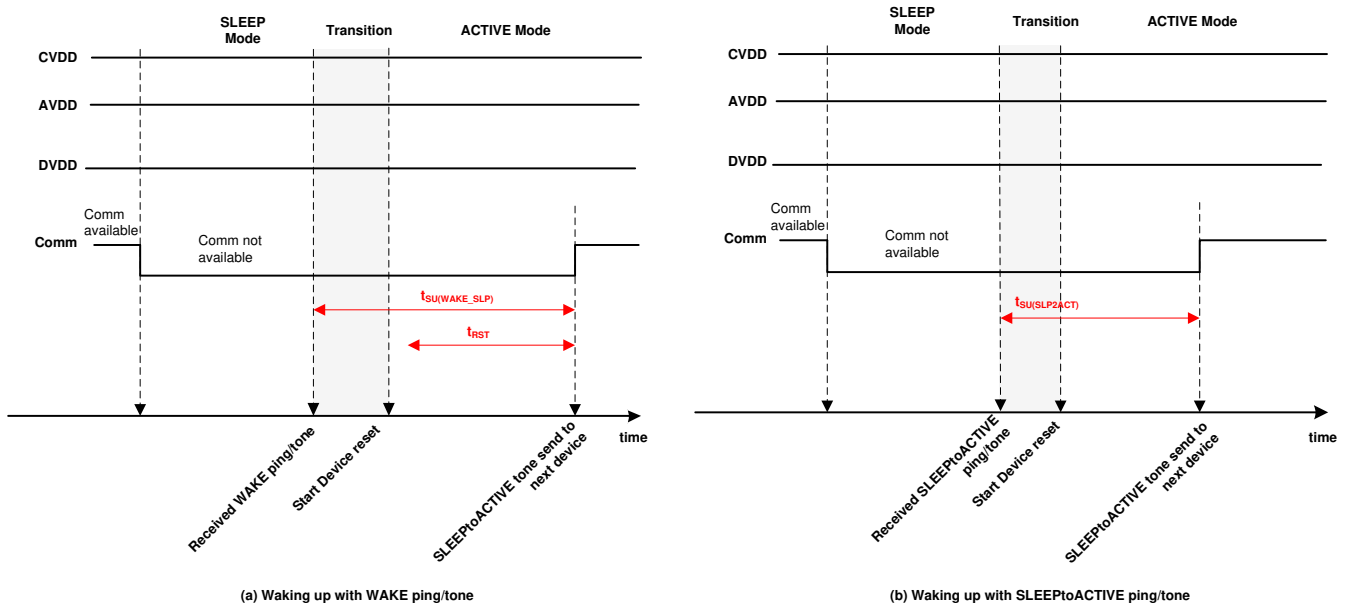
图 7-58. SLEEP 至 ACTIVE 模式转换
