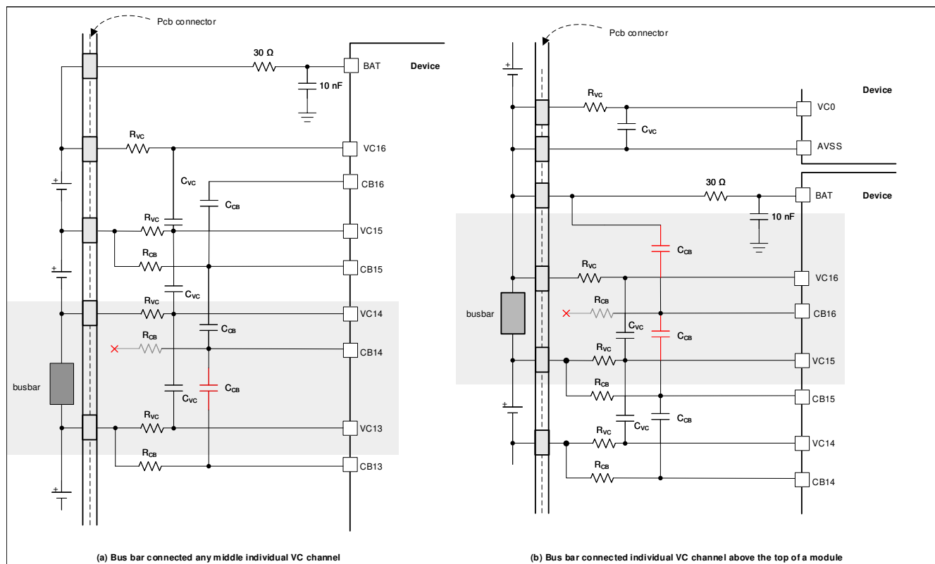
图 7-53. 连接到单个 VC 通道的汇流条
