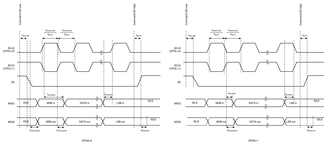
图 7-42. SPI 主器件时序图
