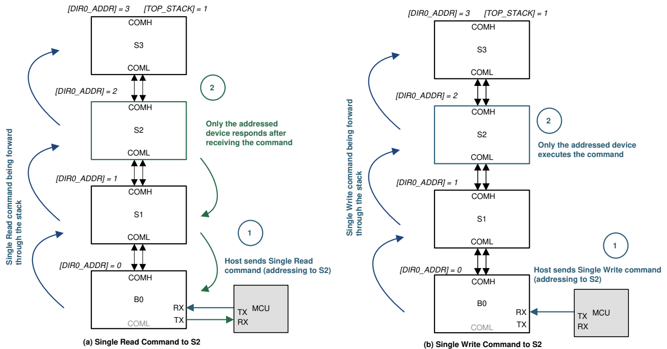
图 7-29. 单器件读取/写入
