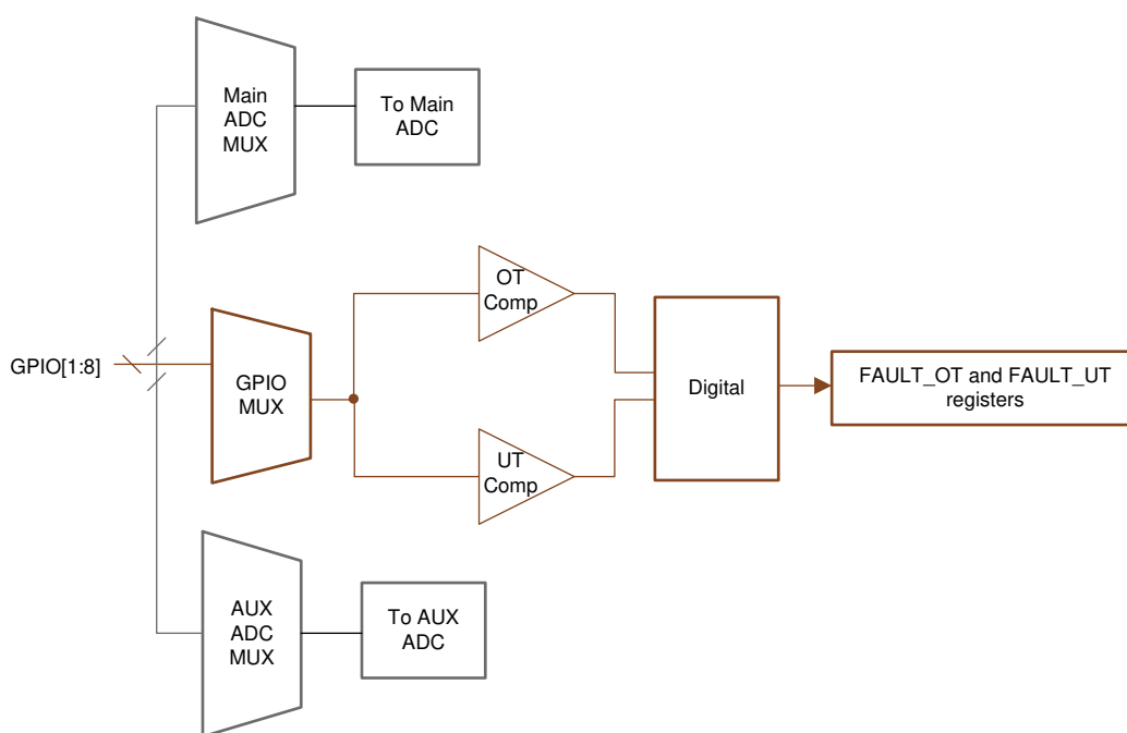
图 7-22. OT 和 UT 保护器
