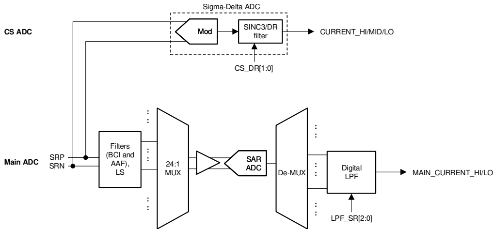
图 7-12. CS ADC
