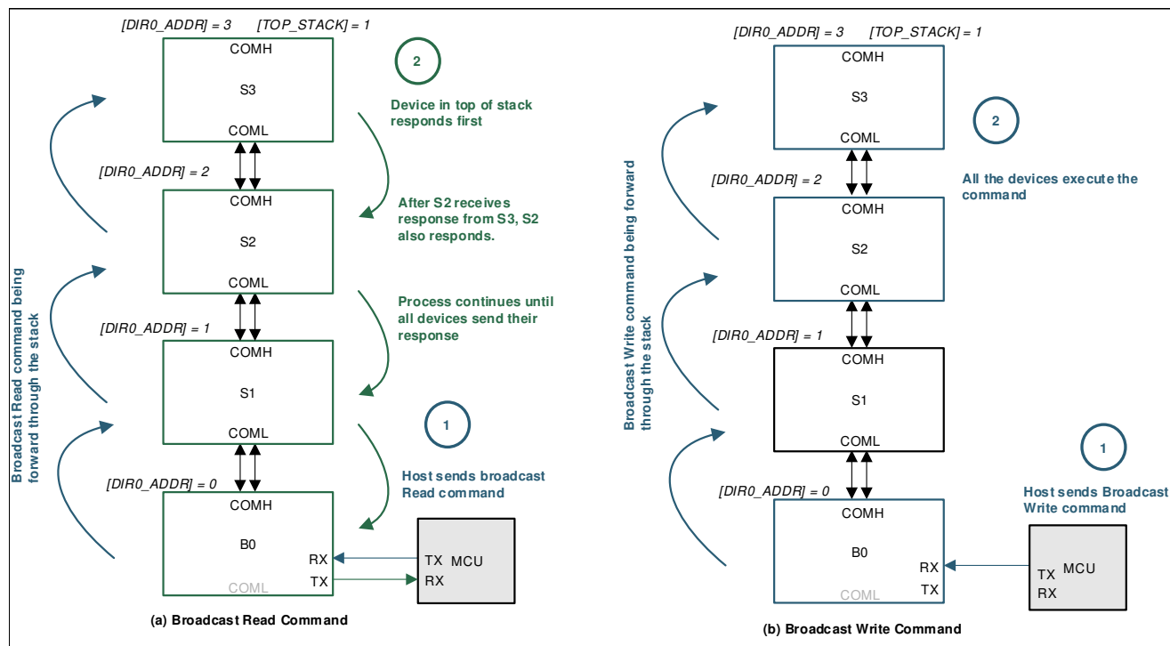
图 7-31. 广播读取/写入
