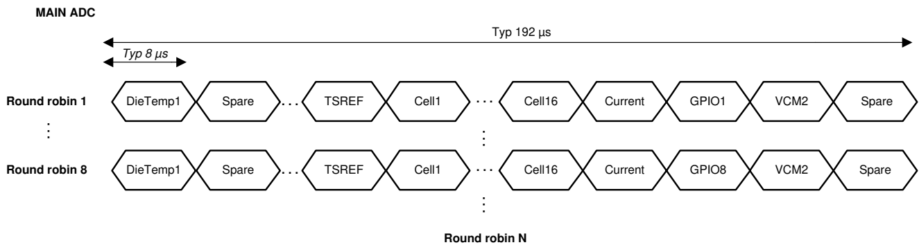
图 7-3. 主 ADC 轮询测量
