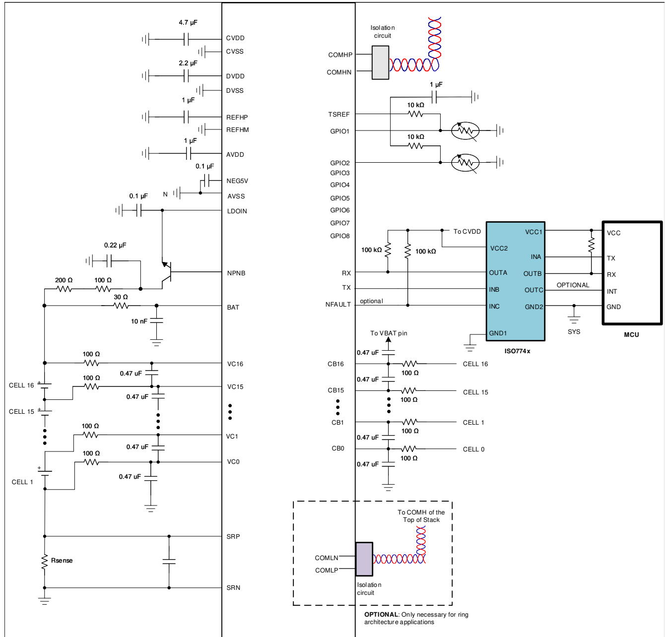
图 8-1. 具有 16S 配置的典型应用电路
