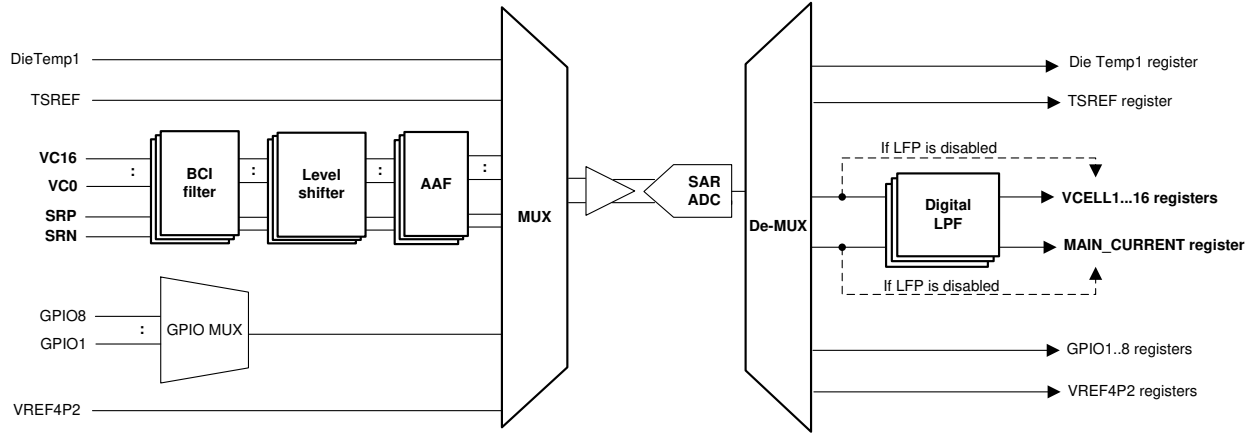
图 7-2. 主 ADC 测量路径
