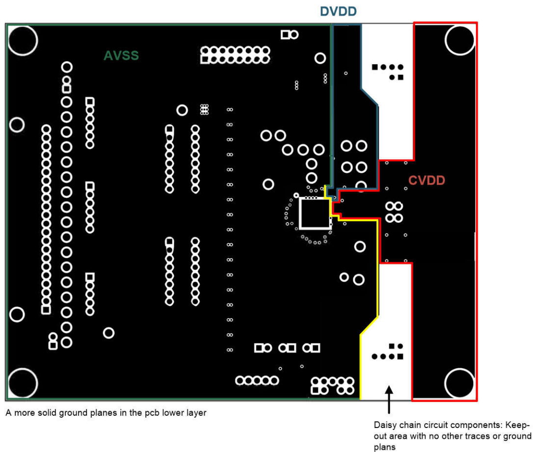
图 10-5. 具有实心独立接地平面的第二层
