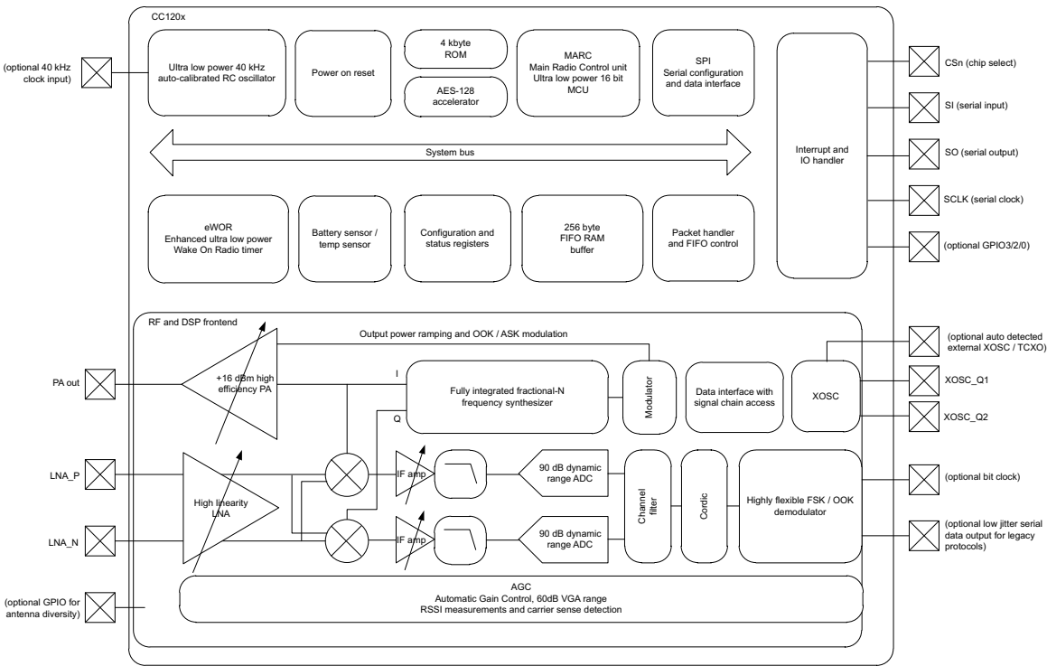
图 1-1. 系统方框图
