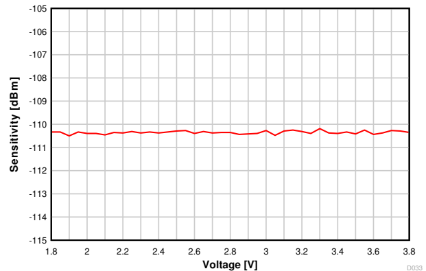
图 7-14. 灵敏度与电源电压 (VDD) 间的关系 ( 50kbps , 868.3MHz )
