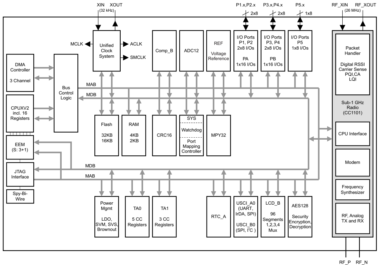
图 1-1. CC430F613x 功能方框图
