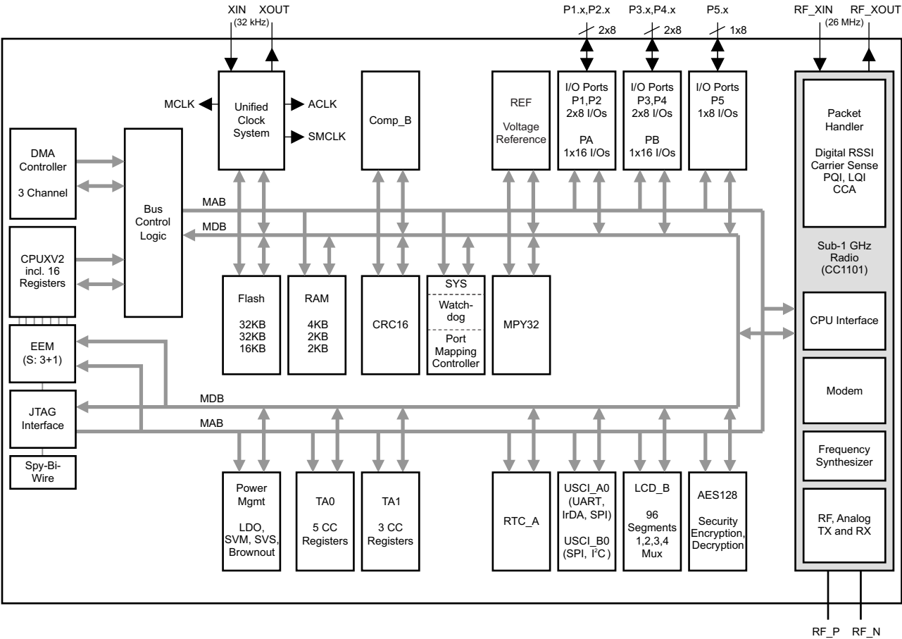
图 1-2. CC430F612x 功能方框图
