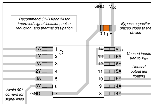
图 7-1. Layout Diagram
