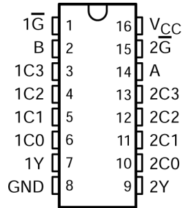
图 3-1. CD54AC153 J 封装，16 引脚 CDIP； CD74AC153 D、N 或 PW 封装；16 引脚 SOIC、PDIP 或 TSSOP（顶视图）
