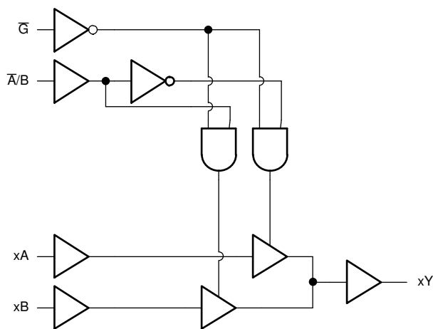
逻辑图
