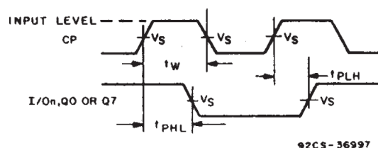
图 5-2. 时钟先决条件和传播延迟
