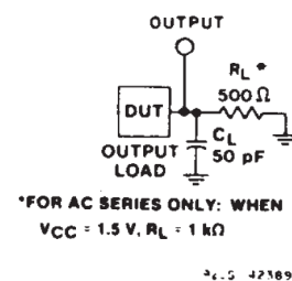
图 5-5. 测试电路
