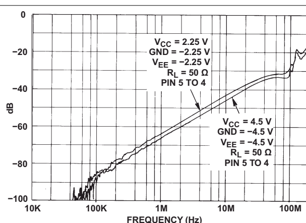
图 5-8. 通道关断带宽 (HC 和 HCT4053)
