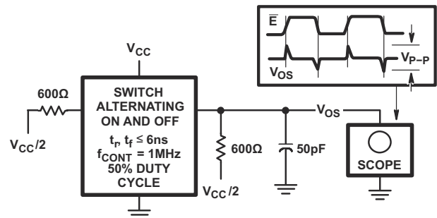
图 6-5. 控制至开关馈通噪声测试电路
