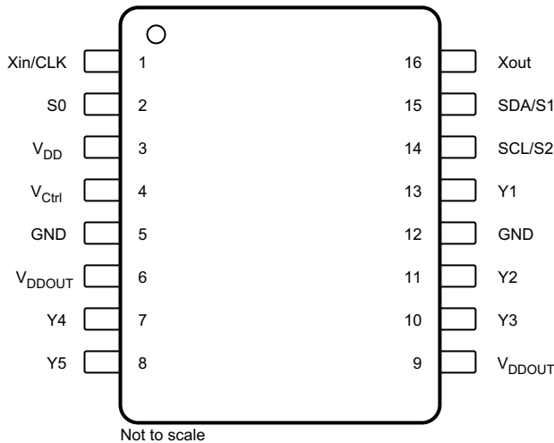
图 4-1. PW 封装 16 引脚 TSSOP 顶视图
