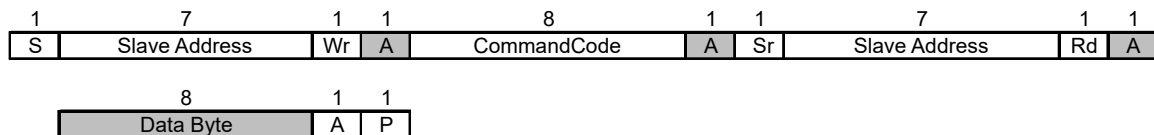
图 7-7. 字节读取协议
