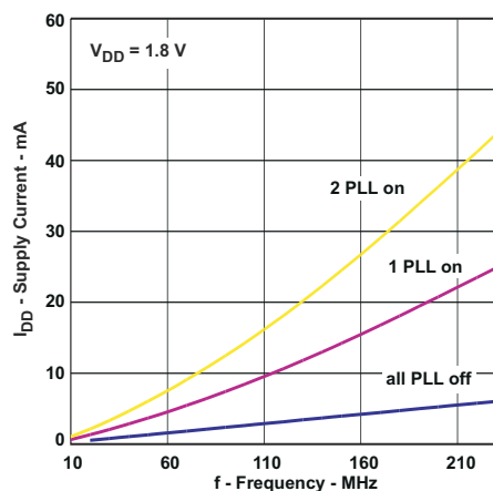
图 5-1. CDCEx925 电源电流与 PLL 频率间的关系
