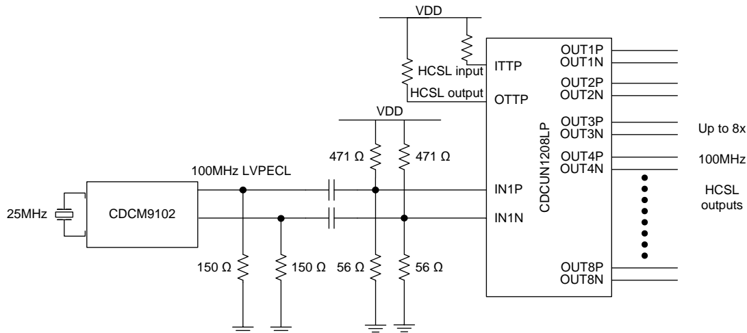
简化电路原理图
