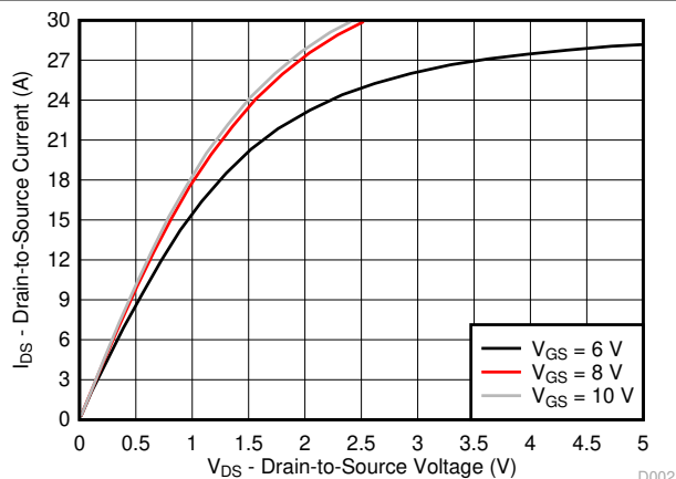
图 4-2. 饱和特性
