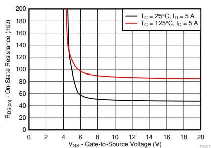
R_{DS(on)} 与 V_{GS} 之间的关系
