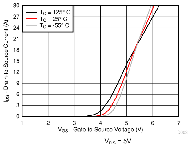
图 4-3. 传输特性
