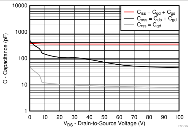
图 4-5. 电容
