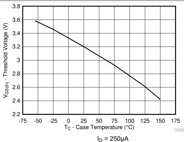
图 4-6. 阈值电压与温度间的关系
