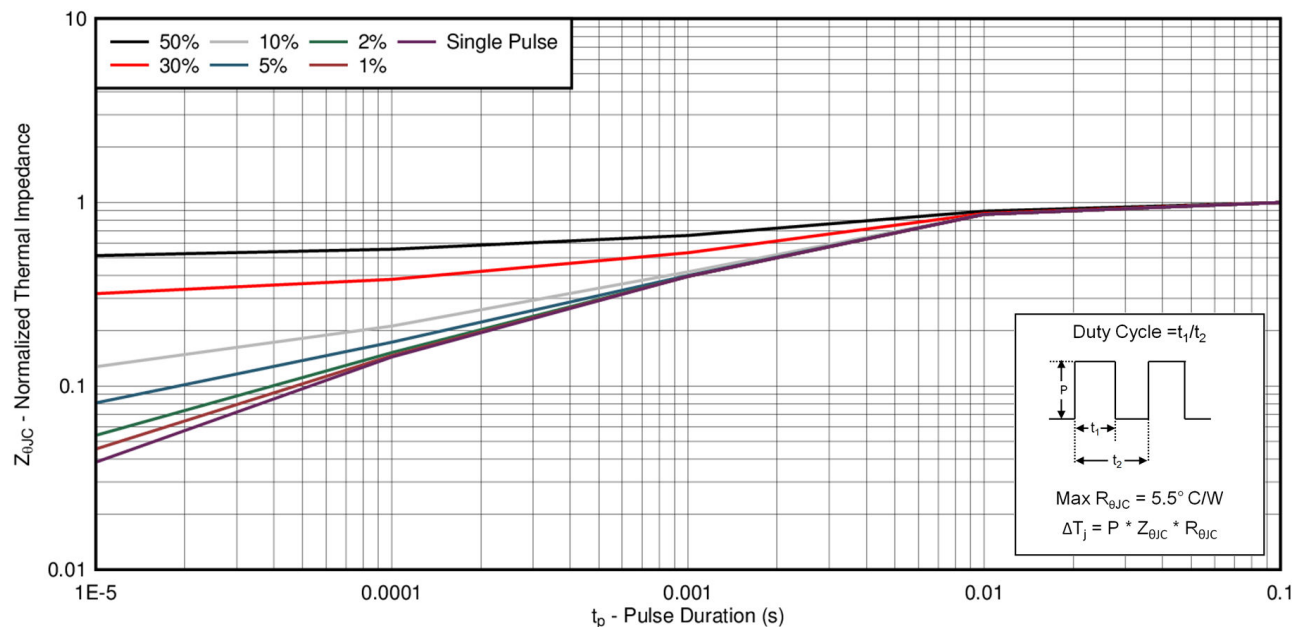
图 4-1. 瞬态热阻抗
