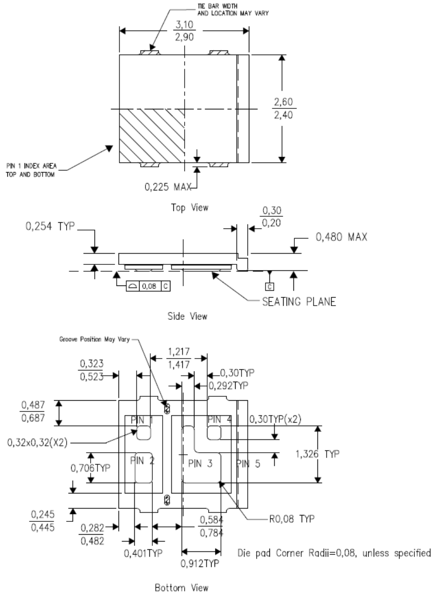
引脚配置
