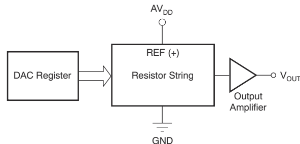
图 8-1. DACx311 Architecture
