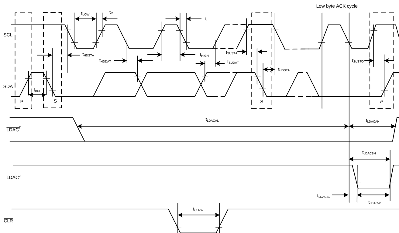
图 1. 串行接口时序图
