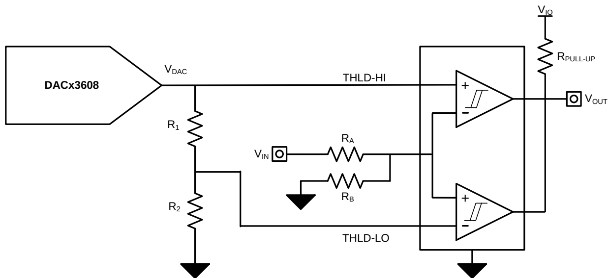
图 66. 可编程窗口比较器
