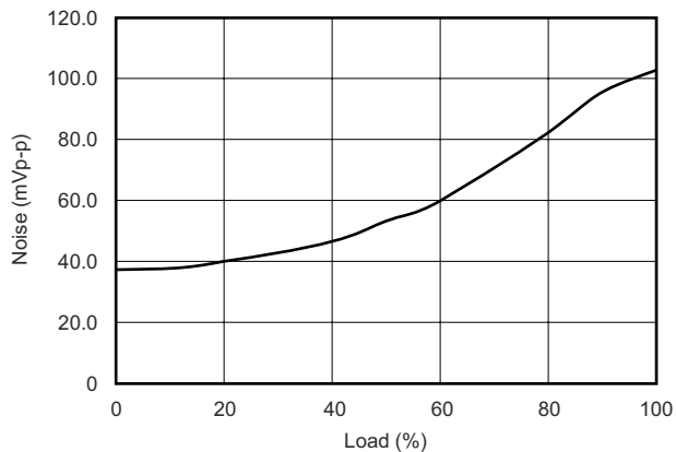
图 7-14. Output Voltage Noise
