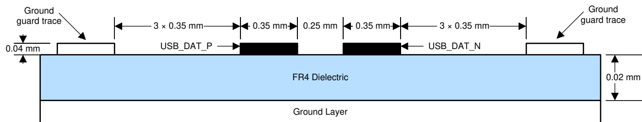
图 9-13. USB Layout Example
