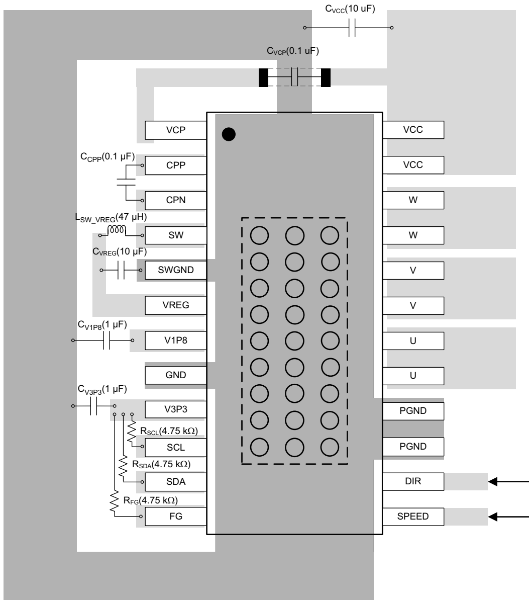
图 43. Layout Schematic
