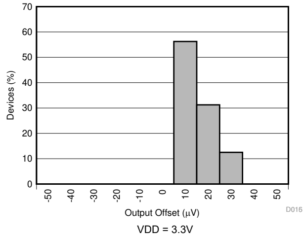
图 5-19. 分流检测放大器输出失调电压柱状图
