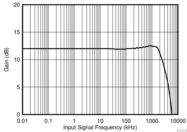
图 5-33. 分流检测放大器增益与输入信号频率间的关系
