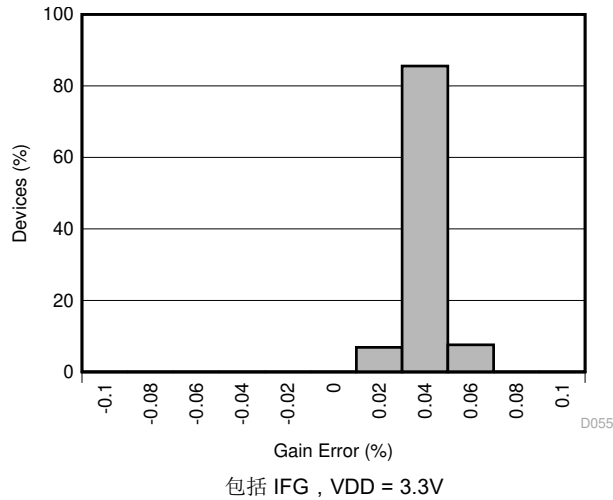
图 5-31. 分流检测放大器增益误差柱状图 包括 IFG, VDD = 3.3V
