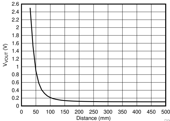
图 7-3. DRV425 的模拟输出电压与磁体距离间的关系
