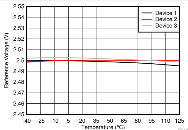
图 5-51. 基准电压与温度间的关系
