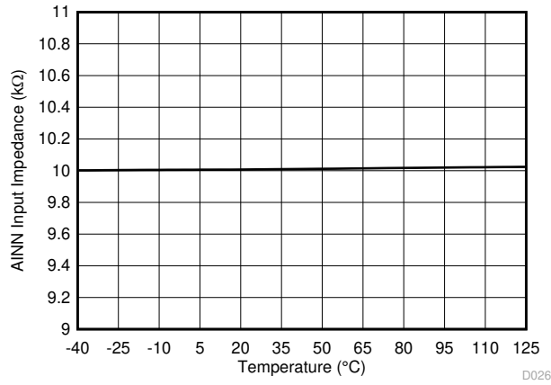
图 5-29. 分流检测放大器 AINN 输入阻抗与温度间的关系
