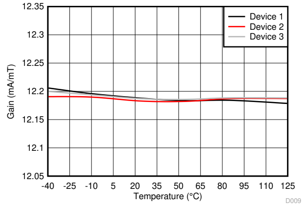
图 5-8. 磁通门传感器前端增益与温度间的关系
