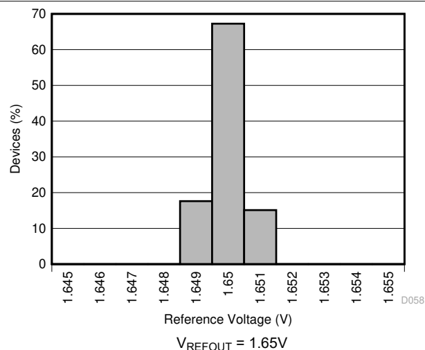
图 5-49. 基准电压柱状图
