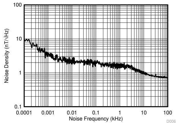
图 5-12. 磁通门传感器前端噪声密度与噪声频率间的关系
