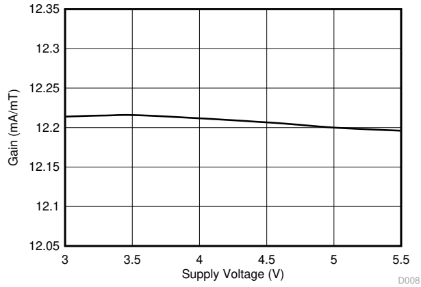
图 5-7. 磁通门传感器前端增益与电源电压间的关系
