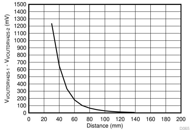
图 7-4. 两个 DRV425 输出之间的差异与磁体距离间的关系
