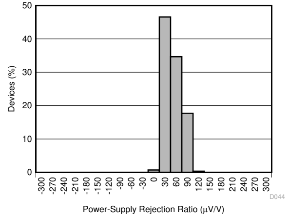
图 5-54. 基准电压 PSRR 柱状图
