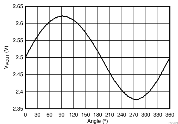
图 6-2. 器件输出与磁场方向间的关系
