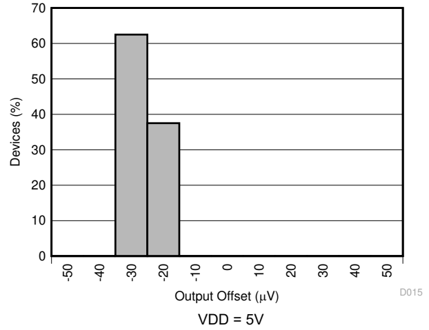
图 5-18. 分流检测放大器输出失调电压柱状图
