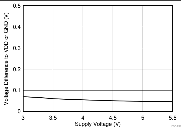
图 5-36. \overline{\text{OR}} 引脚触发电平与电源电压间的关系
