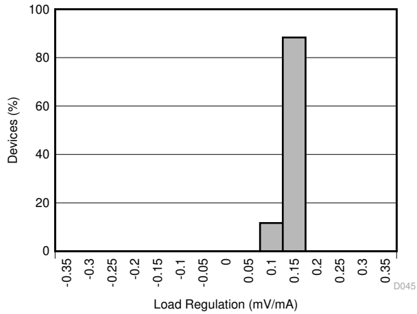
图 5-55. 基准电压负载调整柱状图
