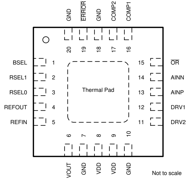
图 4-1. RTJ 封装 20 引脚 WQFN 顶视图
