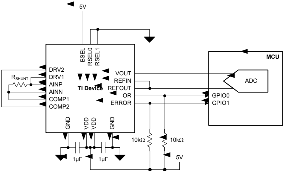
图 7-1. 线性位置检测
