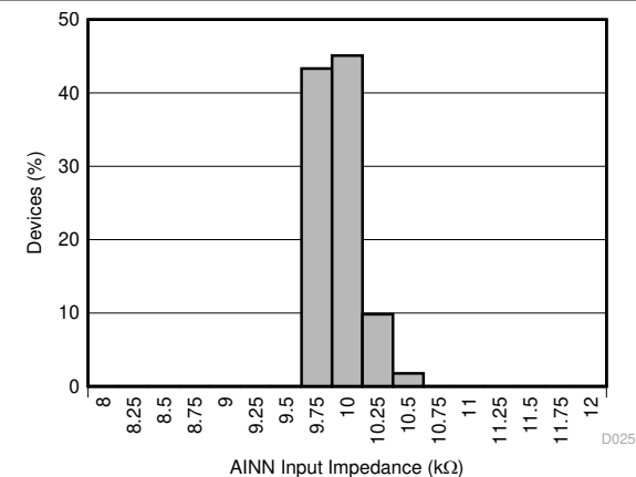
图 5-28. 分流检测放大器 AINN 输入阻抗柱状图
