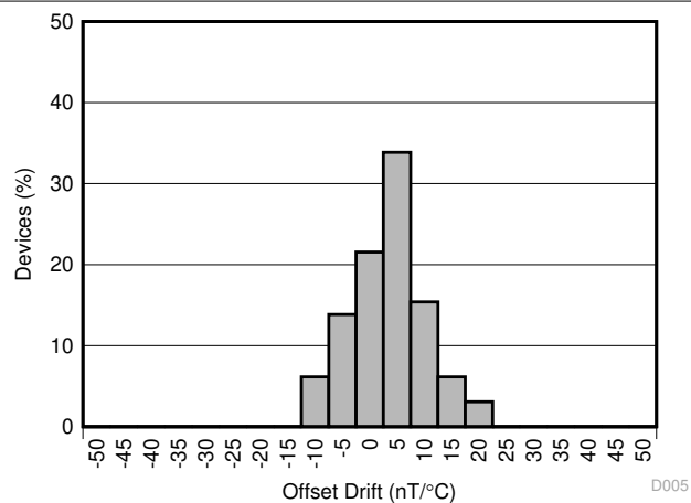
图 5-5. 磁通门传感器前端失调漂移柱状图
