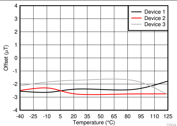
图 5-4. 磁通门传感器前端失调与温度间的关系
