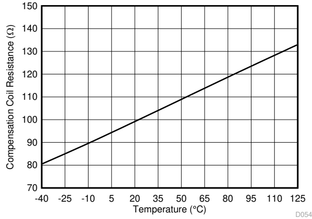
图 5-17. 补偿线圈电阻与温度间的关系
