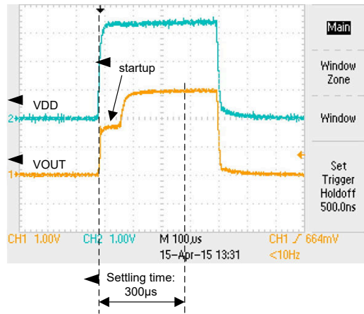
图 6-6. DRV425 VOUT 输出的趋稳时间
