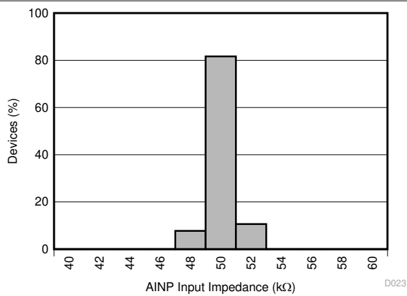
图 5-26. 分流检测放大器 AINP 输入阻抗柱状图
