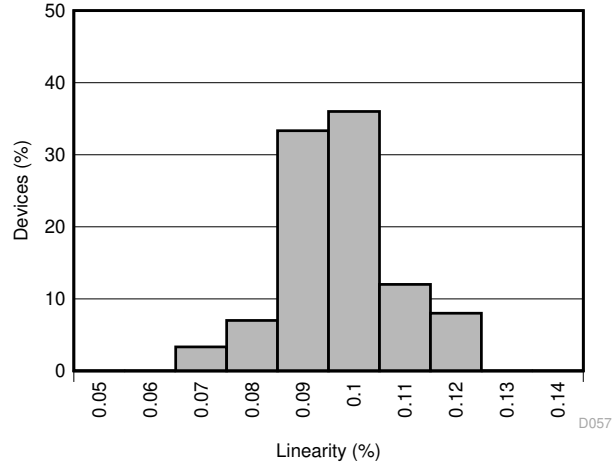
图 5-9. 磁通门传感器前端线性度柱状图
