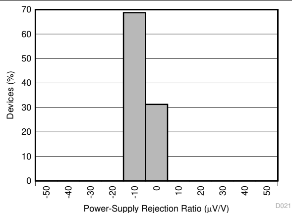
图 5-24. 分流检测放大器 PSRR 柱状图
