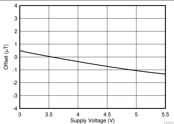
图 5-3. 磁通门传感器前端失调与电源电压间的关系
