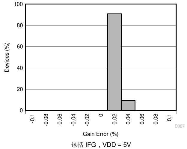
图 5-30. 分流检测放大器增益误差柱状图 包括 IFG, VDD = 5V
