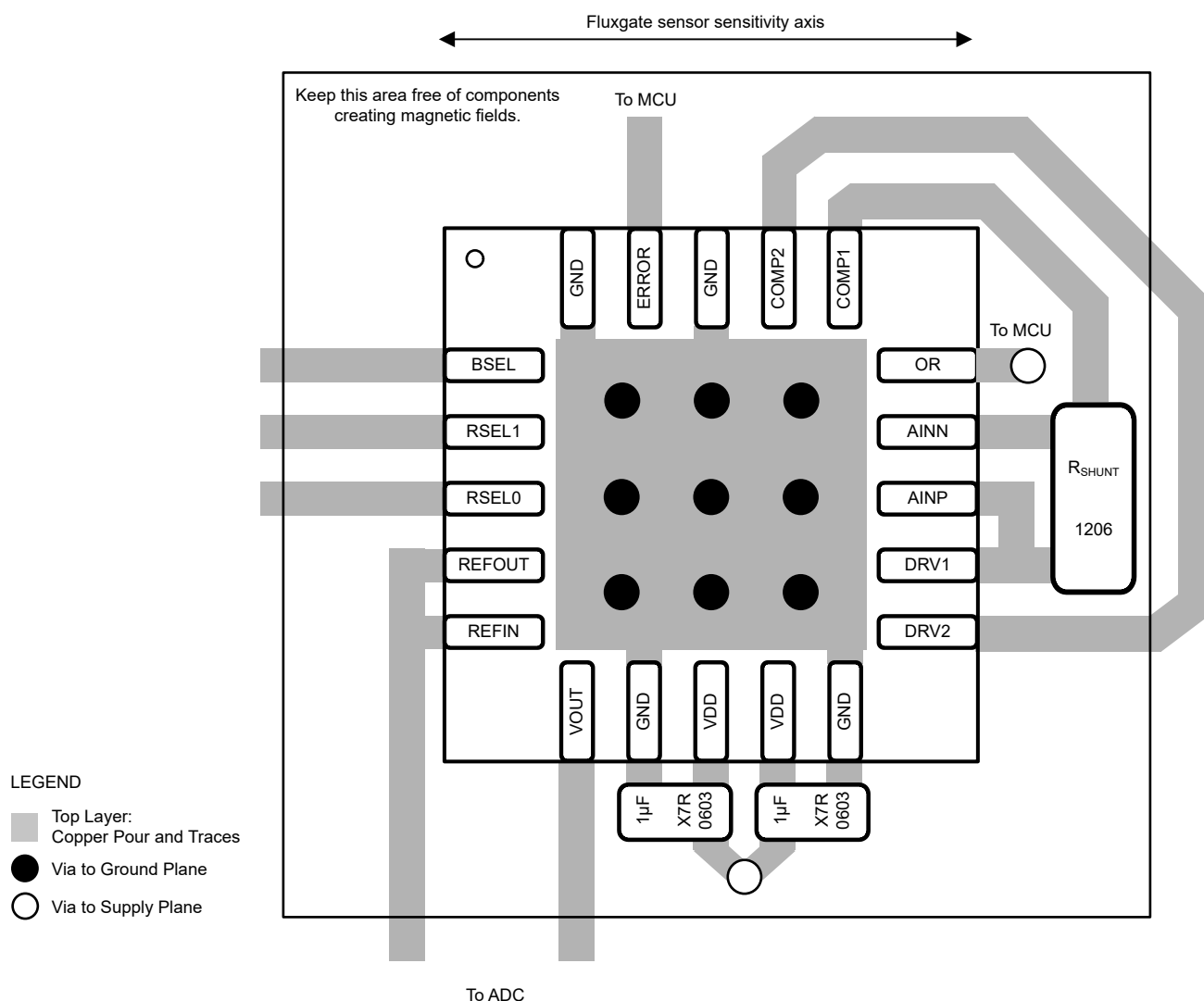
图 7-10. 通用布局示例 ( 顶视图 )
