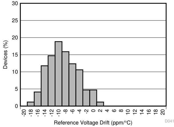
图 5-53. 基准电压漂移柱状图
