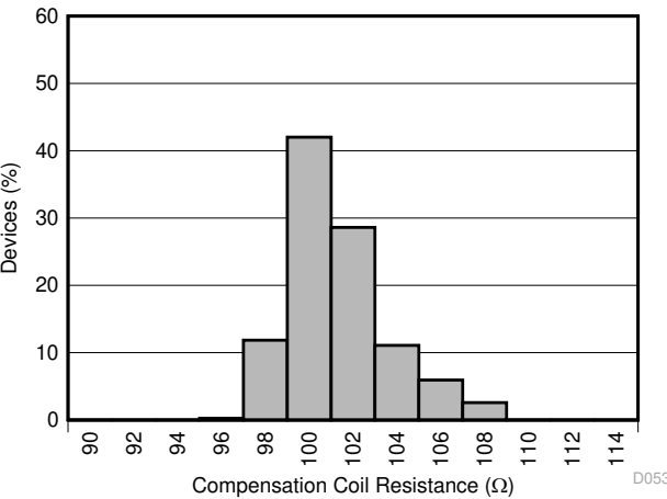
图 5-16. 补偿线圈电阻柱状图
