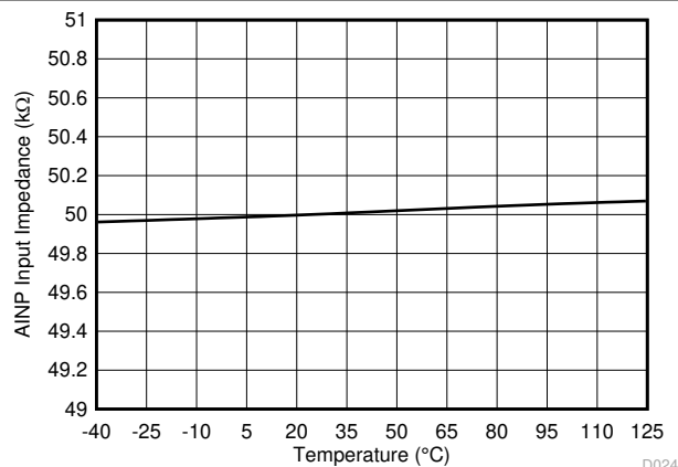
图 5-27. 分流检测放大器 AINP 输入阻抗与温度间的关系
