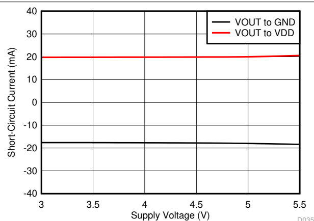
图 5-39. 分流检测放大器输出短路电流与电源电压间的关系
