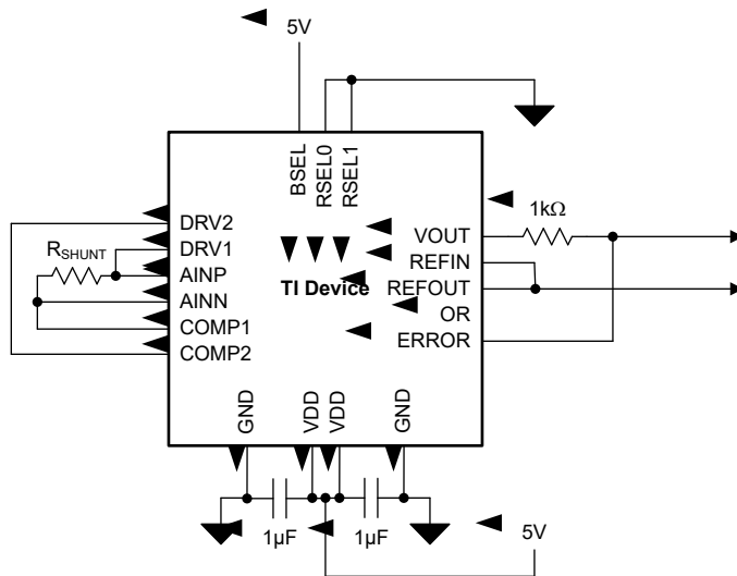
图 6-4. 使用 VOUT 和 ERROR 引脚组合进行磁场超范围检测
