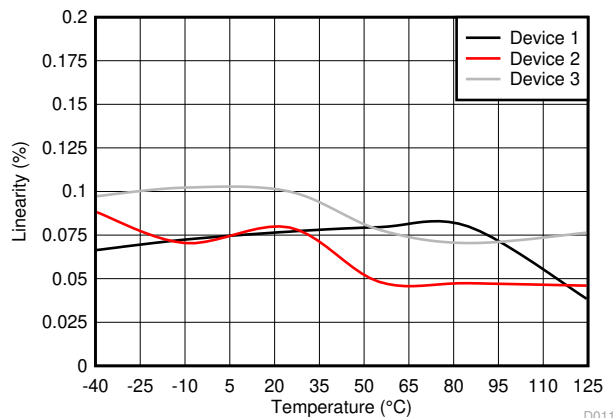
图 5-11. 磁通门传感器前端线性度与温度间的关系
