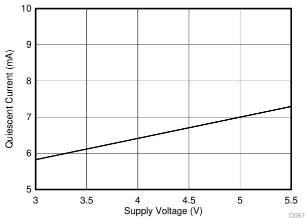
图 5-57. 静态电流与电源电压间的关系
