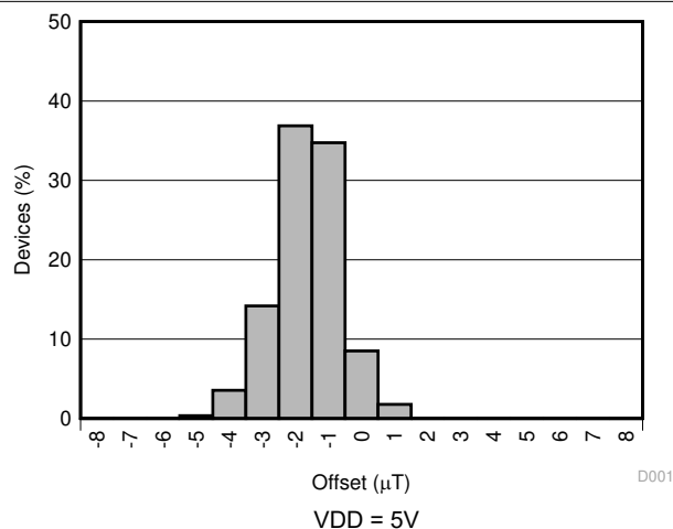
图 5-1. 磁通门传感器前端失调柱状图
