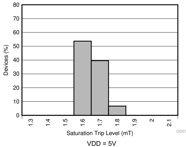
图 5-13. 磁通门传感器饱和 ( \overline{\text{ERROR}} 引脚 ) 触发电平柱状图
