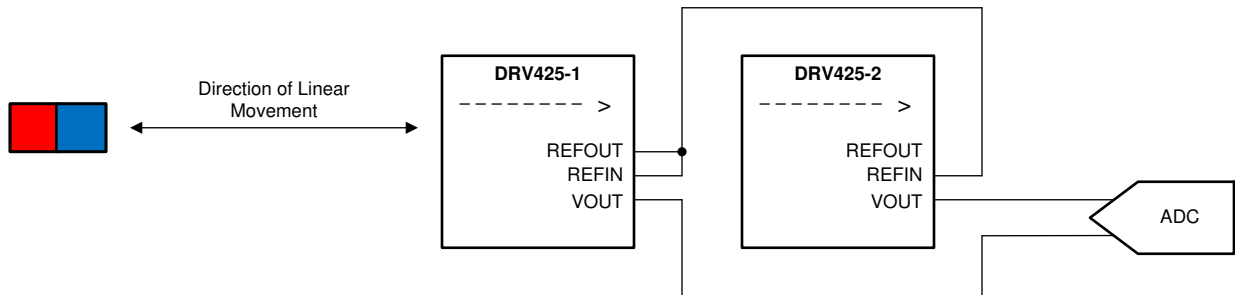
图 7-2. 采用两个 DRV425 器件的差分线性位置检测
