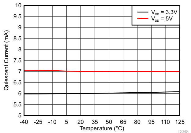
图 5-58. 静态电流与温度间的关系
