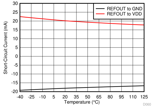
图 5-56. 基准短路电流与温度间的关系
