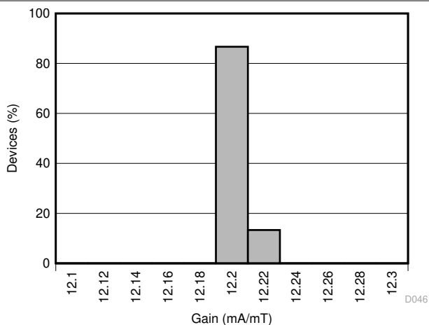
图 5-6. 磁通门传感器前端增益柱状图
