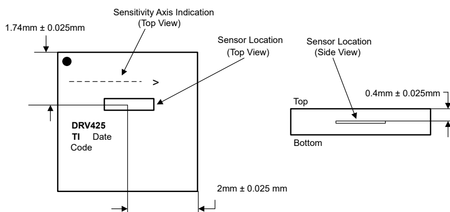
图 6-1. 集成式磁通门传感器的磁性灵敏度方向
