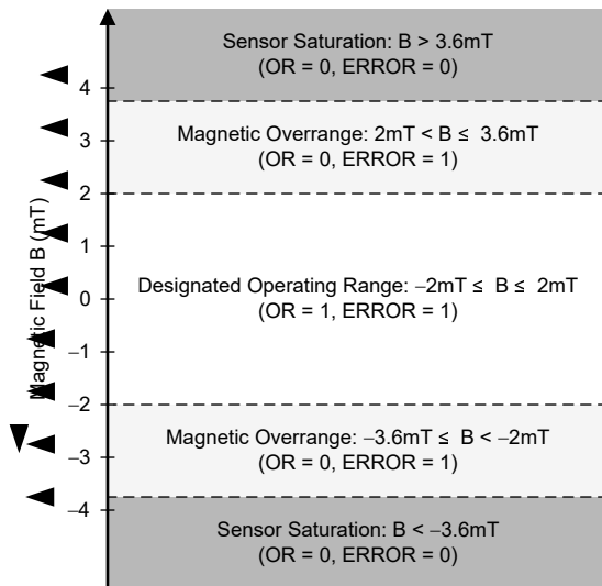
图 6-3. DRV425 的磁场范围 (VDD = 5V 且 R SHUNT = 22 Ω)
