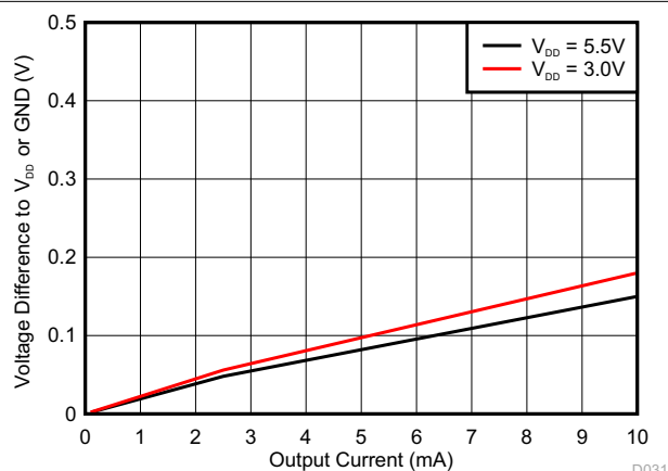
图 5-35. \overline{\text{OR}} 引脚触发电平与输出电流间的关系
