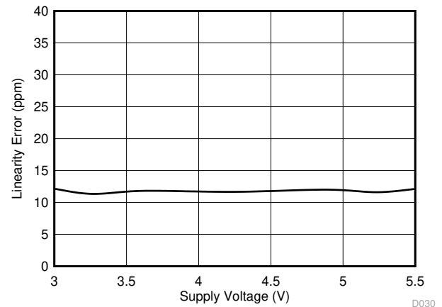
图 5-34. 分流检测放大器线性误差与电源电压间的关系
