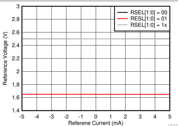
图 5-52. 基准电压与基准输出电流间的关系
