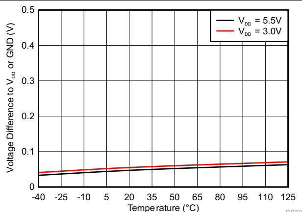
图 5-37. \overline{\text{OR}} 引脚触发电平与温度间的关系
