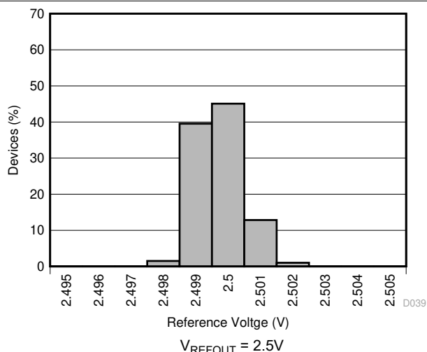
图 5-48. 基准电压柱状图
