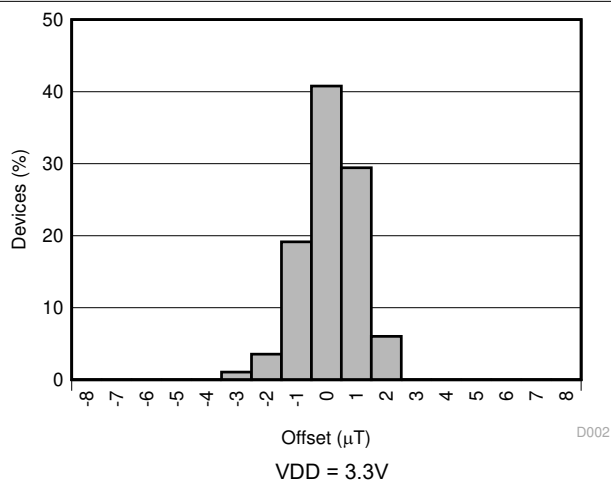
图 5-2. 磁通门传感器前端失调柱状图
