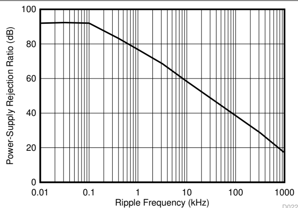
图 5-25. 分流检测放大器 PSRR 与纹波频率间的关系
