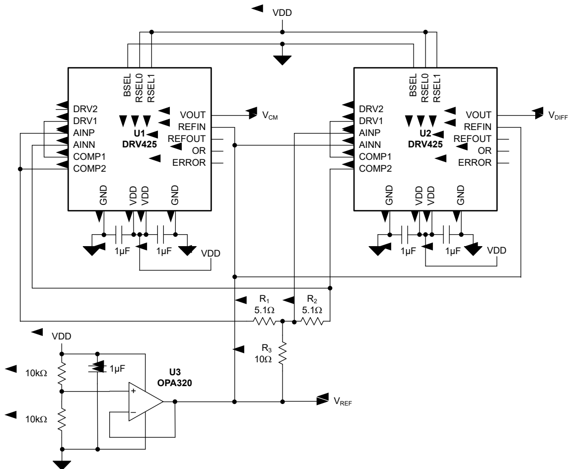
图 7-7. 母线电流检测电路
