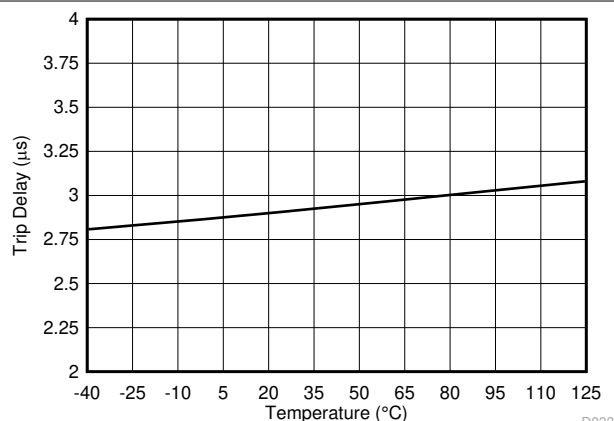
图 5-38. \overline{\text{OR}} 引脚触发延迟与温度间的关系
