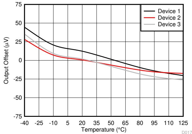
图 5-21. 分流检测放大器输出失调电压与温度间的关系
