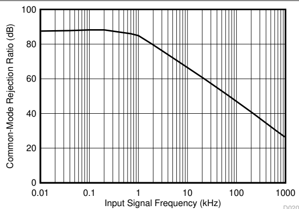
图 5-23. 分流检测放大器 CMRR 与输入信号频率间的关系
