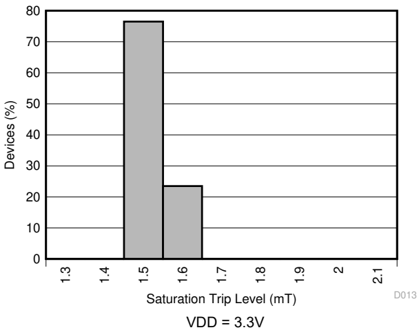
图 5-14. 磁通门传感器饱和 ( \overline{\text{ERROR}} 引脚 ) 触发电平柱状图
