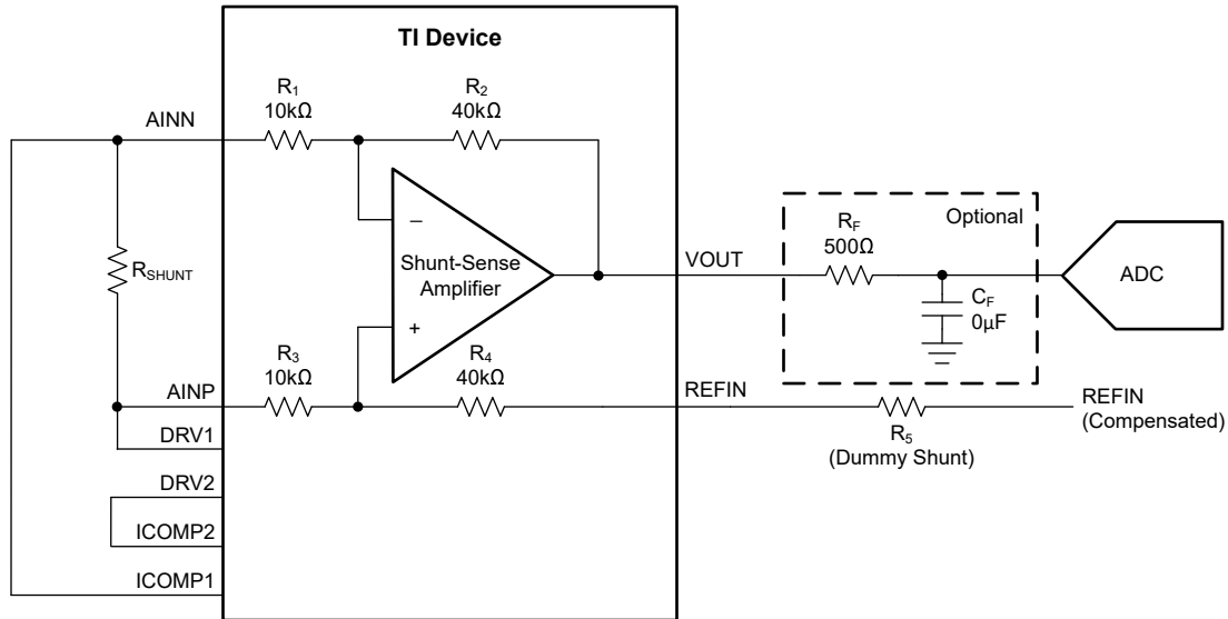
图 6-5. 带有去耦滤波器示例的内部差分放大器
