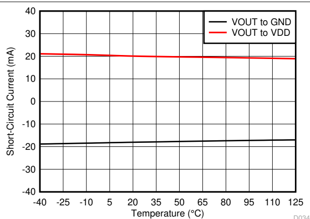
图 5-40. 分流检测放大器输出短路电流与温度间的关系
