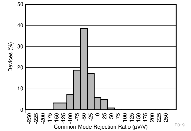
图 5-22. 分流检测放大器 CMRR 柱状图
