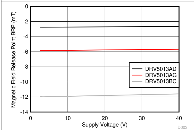
T_A = 25^\circ\text{C} 图 6-5. B_{RP} 与 V_{CC} 之间的关系
