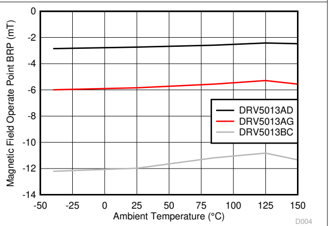
V_{CC} = 3.3\text{V} 图 6-6. B_{RP} 与温度之间的关系
