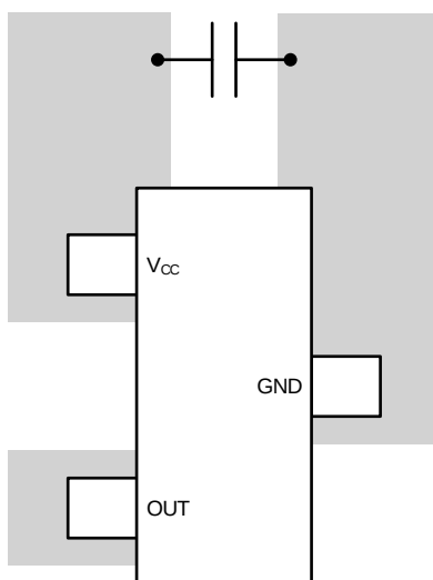
图 23. Example Layout
