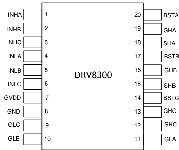
图 6-1. DRV8300-Q1 PW Package 20-Pin TSSOP Top View
