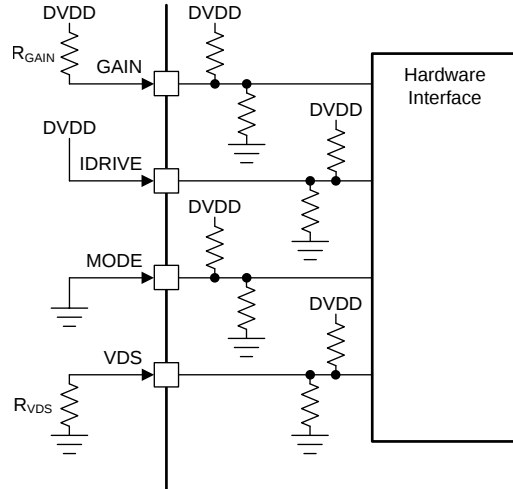
图 18. Hardware Interface
