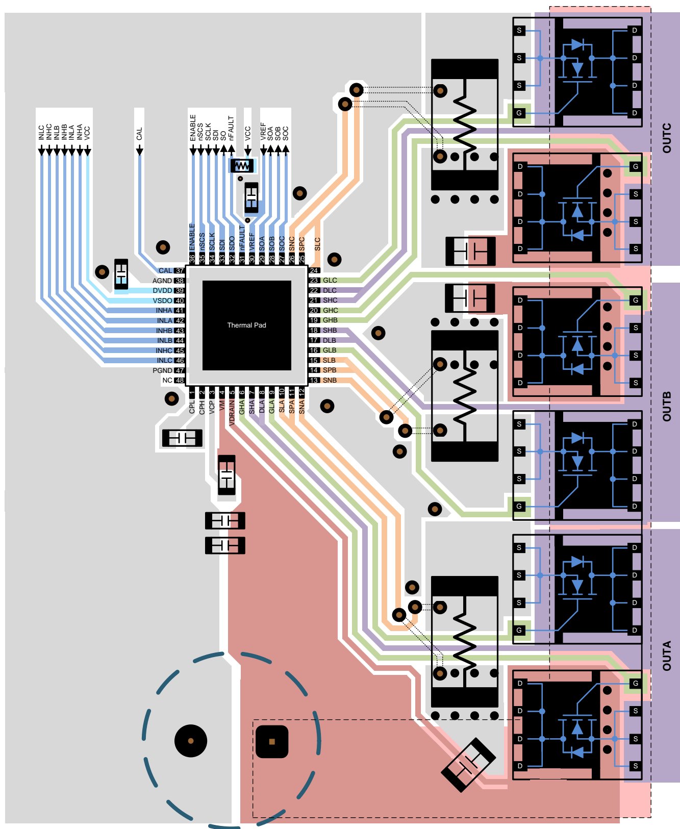
图 69. Layout Example
