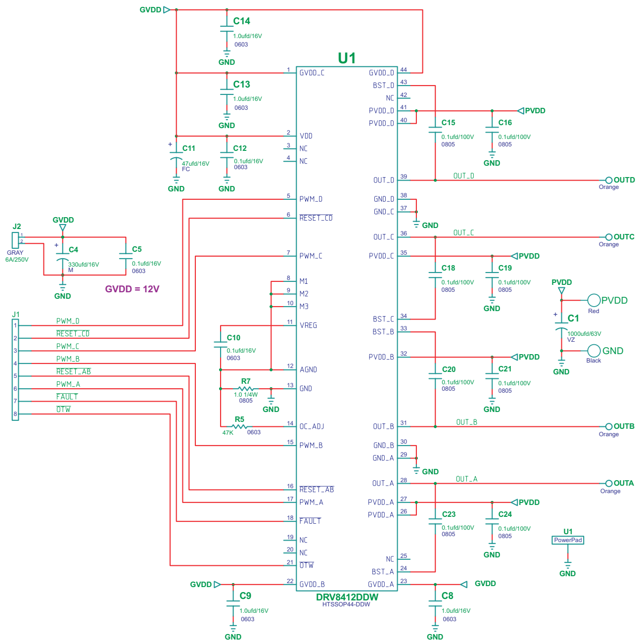
图 7-13. DRV8412 Schematic Example
