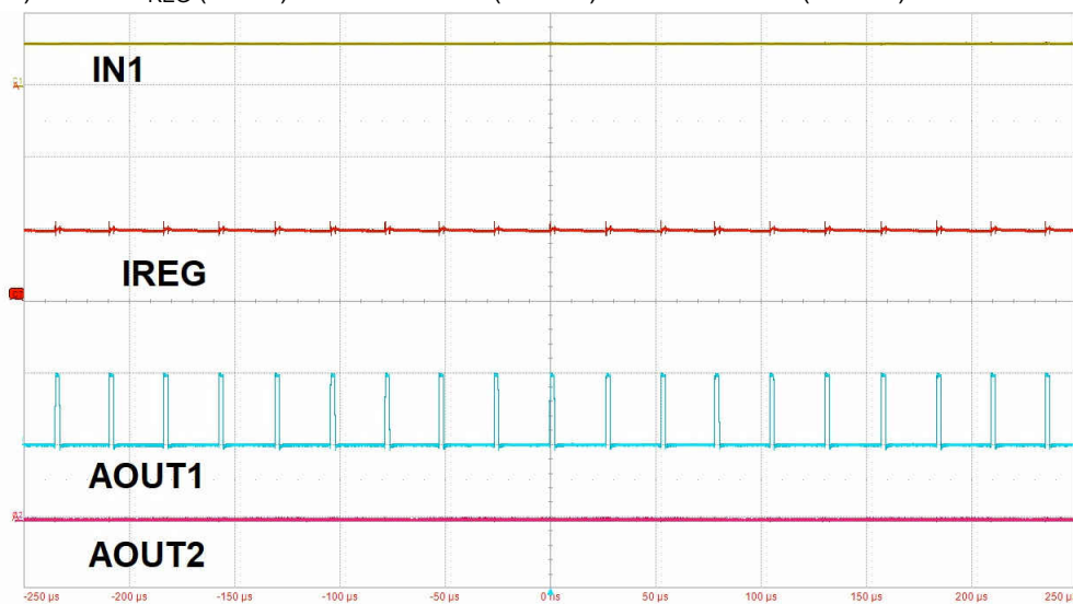
图 8-4. 在进行电流调节的情况下，驱动器全开运行
