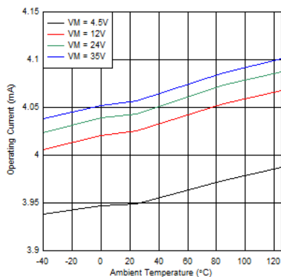
图 6-4. 工作电流与温度之间的关系
