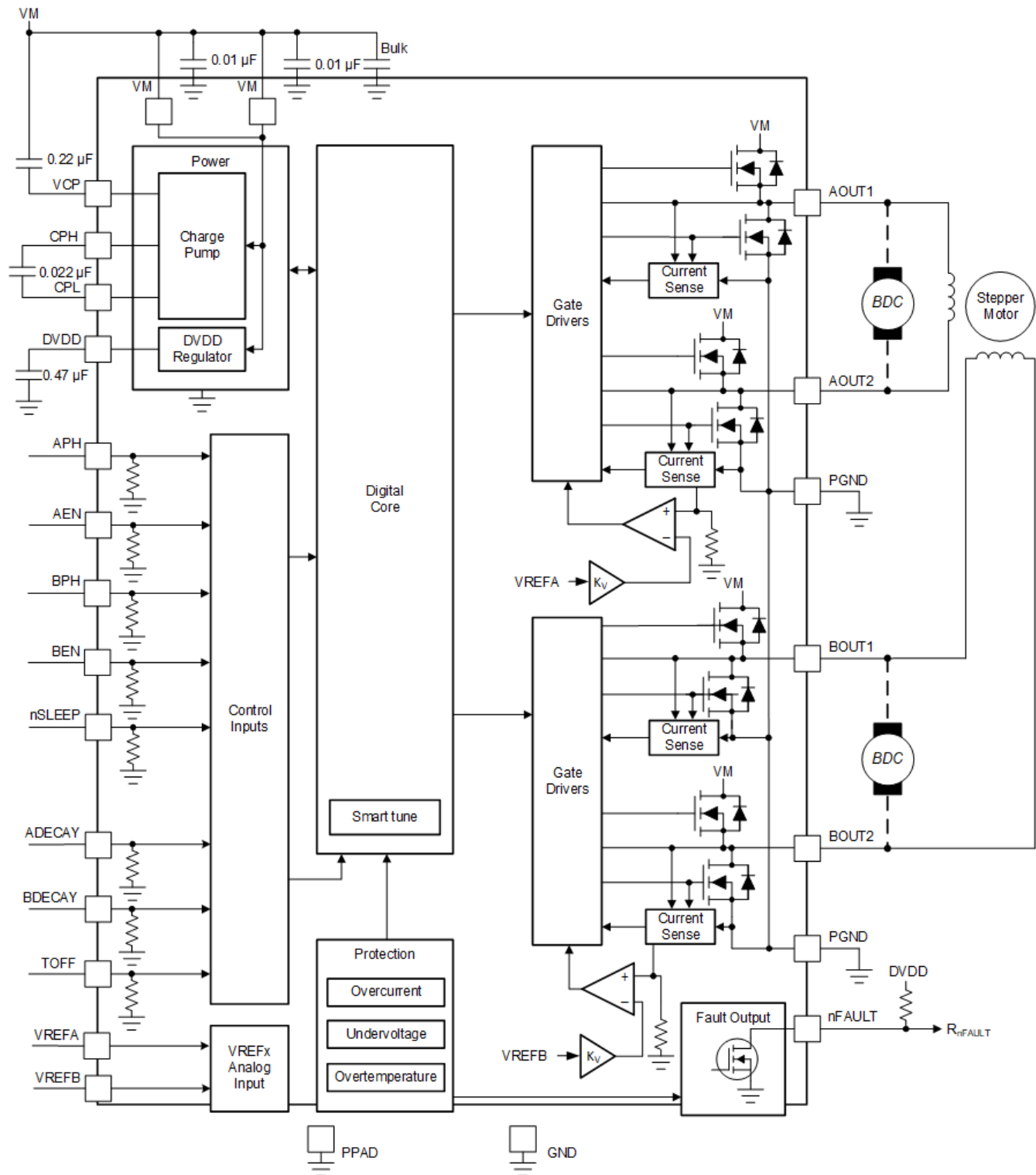
图 7-1. DRV8426E 方框图
