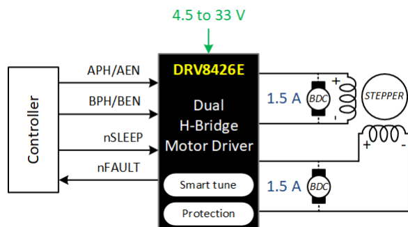
DRV8426E 简化原理图
