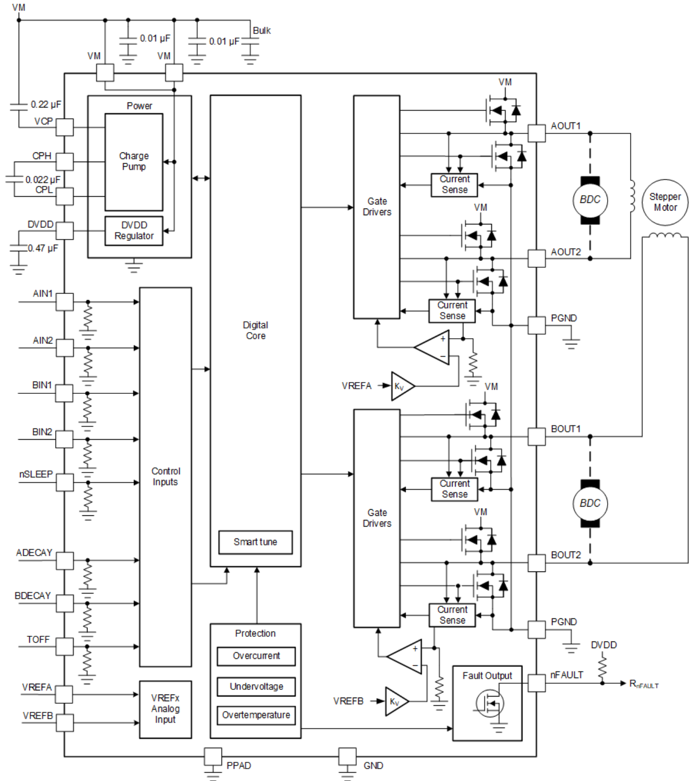
图 7-2. DRV8426P 方框图
