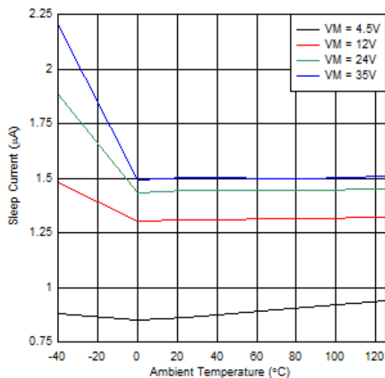
图 6-2. 睡眠电流与温度之间的关系
