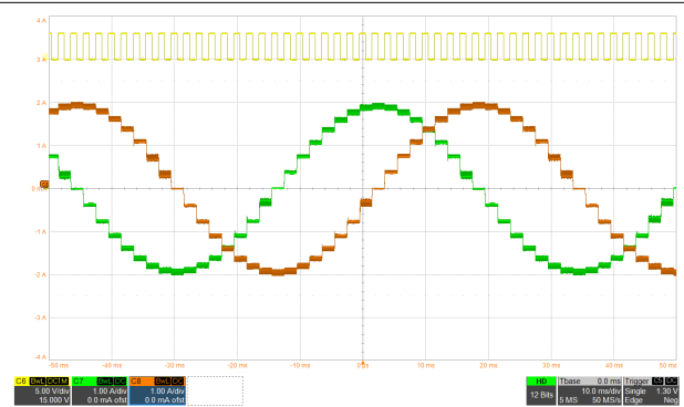
图 8-4. 智能调优动态衰减下的 1/8 微步进
