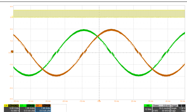
图 8-6. 智能调优动态衰减下的 1/32 微步进
