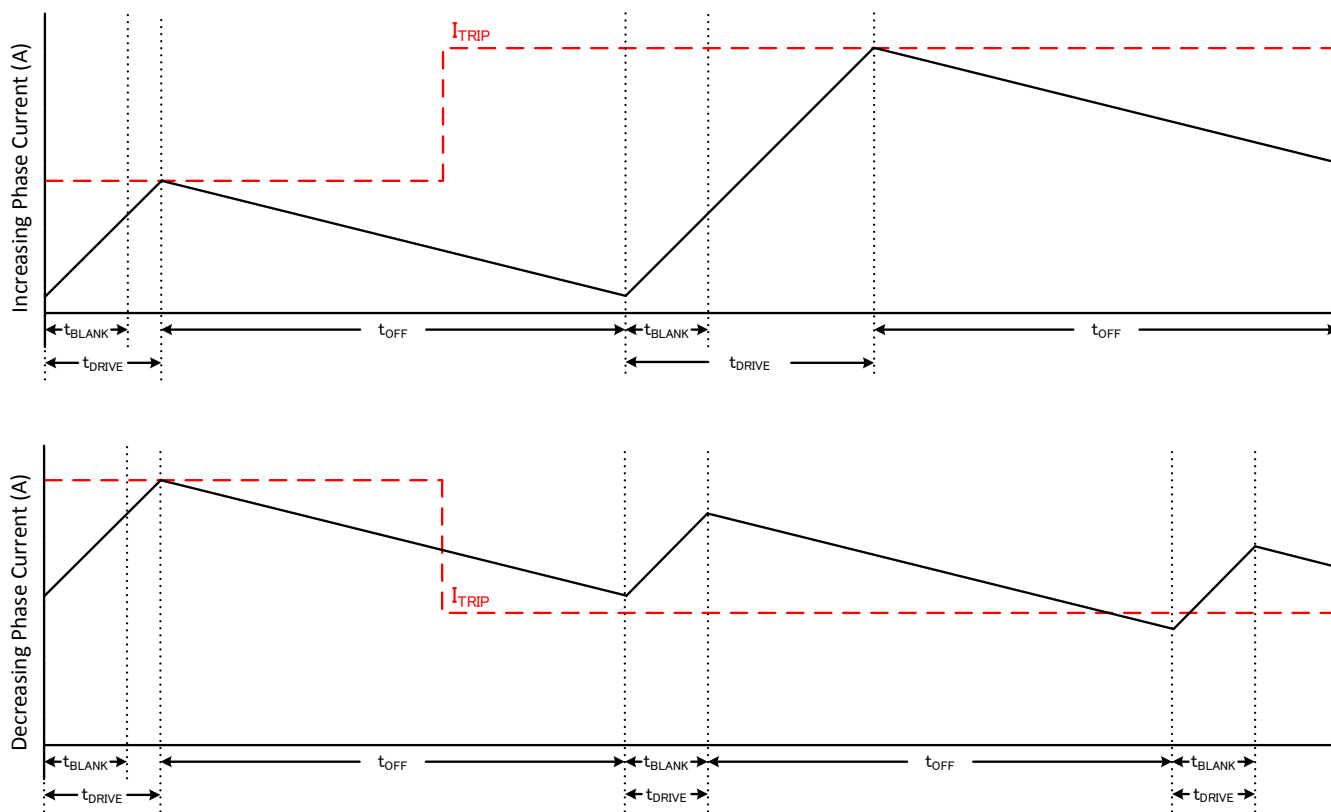
图 7-8. Slow/Slow Decay Mode
