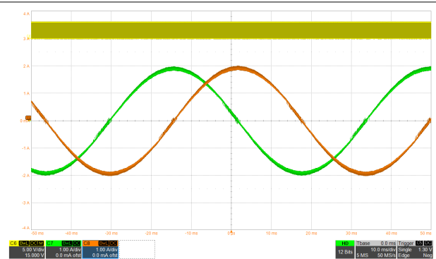
图 8-8. 智能调优动态衰减下的 1/256 微步进
