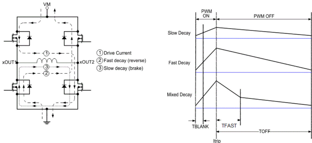
图 7-6. Decay Modes
