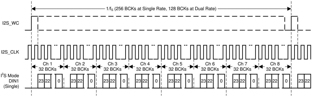
图 8-9. TDM 格式
