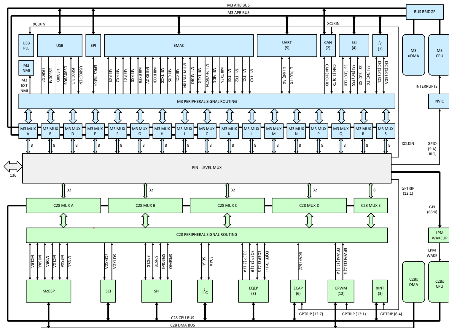
图 6-15. GPIO_MUX1 Block
