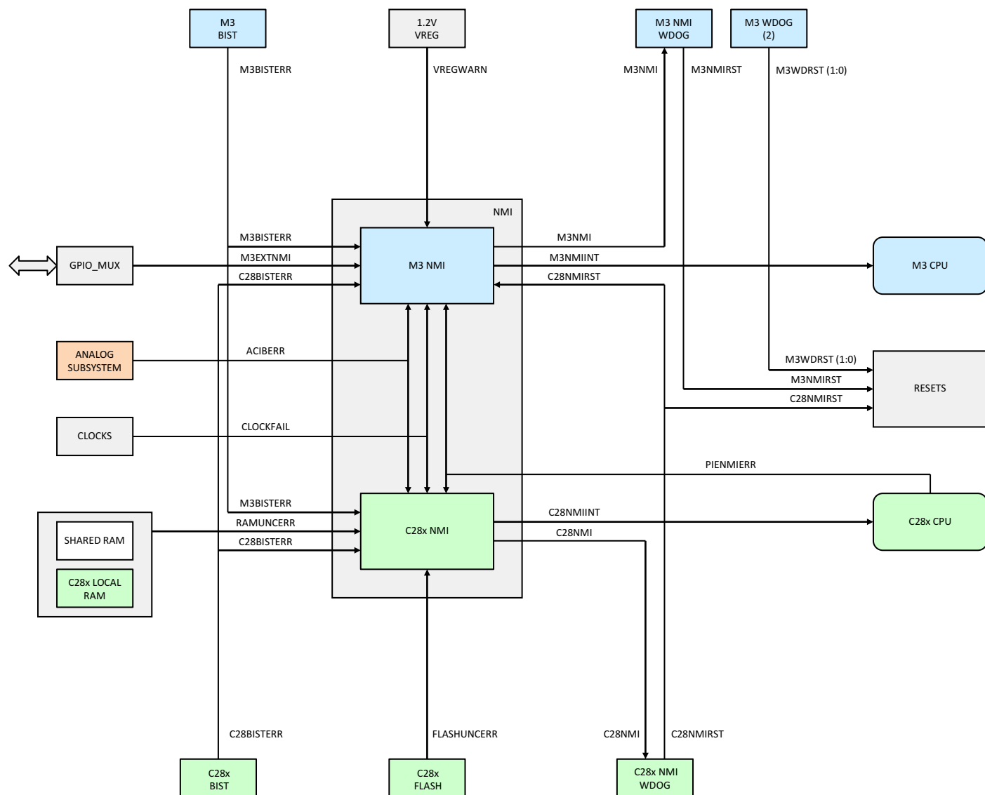
图 6-4. Cortex-M3 NMI and C28x NMI
