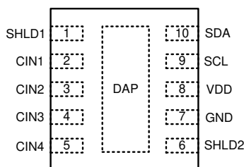
图 4-1. WSON (DSC) 10 Pins TOP
