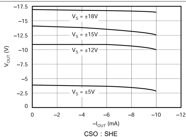
图 5-7. 最大 V_{OUT} 与 I_{OUT} 间的关系 (负摆幅)
