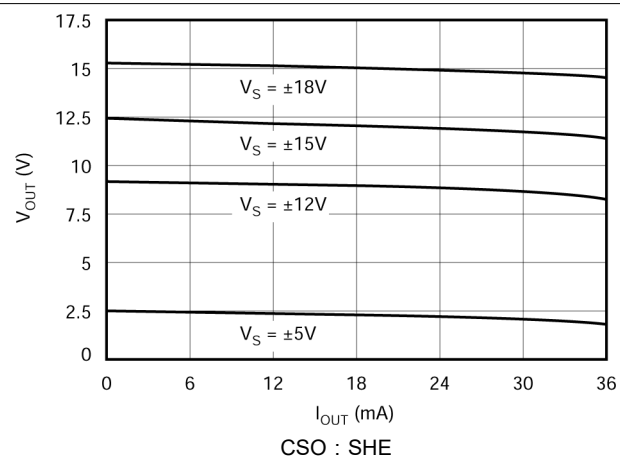
图 5-9. 最大 V_{OUT} 与 I_{OUT} 间的关系 (正摆幅)
