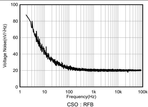
图 5-14. 电压噪声密度与频率间的关系
