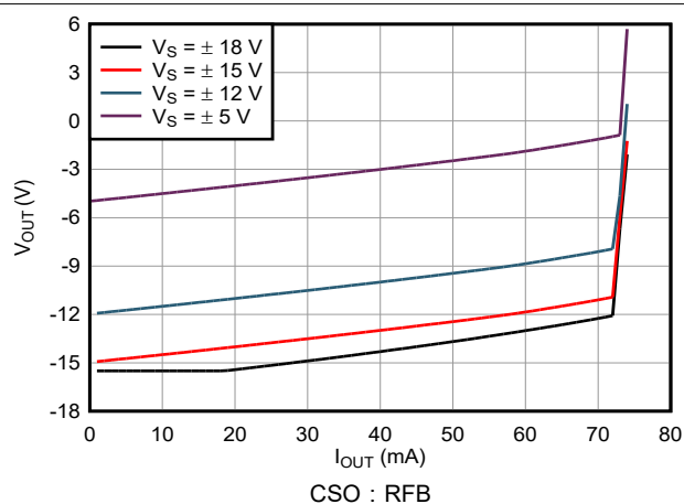
图 5-10. 最大 V_{OUT} 与 I_{OUT} 间的关系 (正摆幅)
