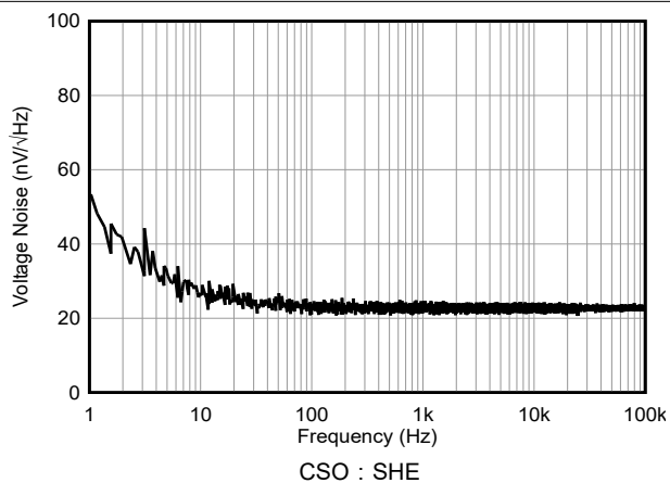
图 5-13. 电压噪声密度与频率间的关系
