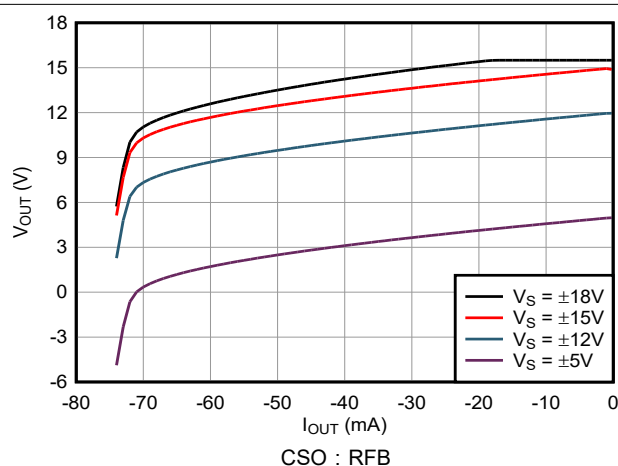
图 5-8. 最大 V_{OUT} 与 I_{OUT} 间的关系 (负摆幅)
