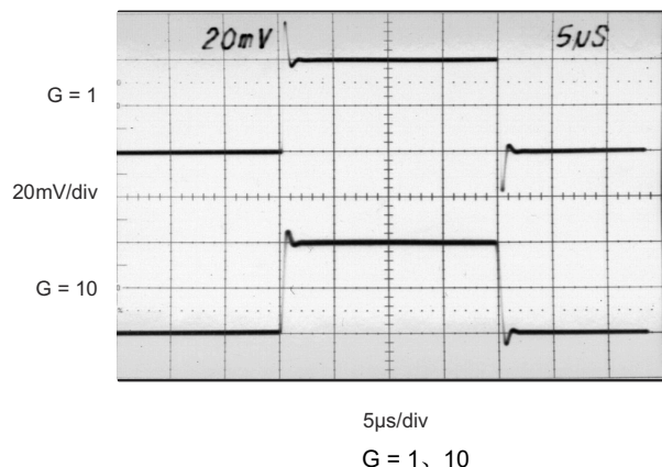
图 8-4. 小信号
