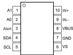
图 5-2. DGS Package 10-Pin VSSOP (Top View)
