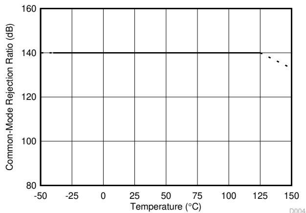
图 5-4. Shunt Input CMRR vs Temperature
