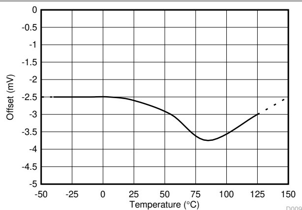
图 5-9. Bus Input Offset Voltage vs Temperature
