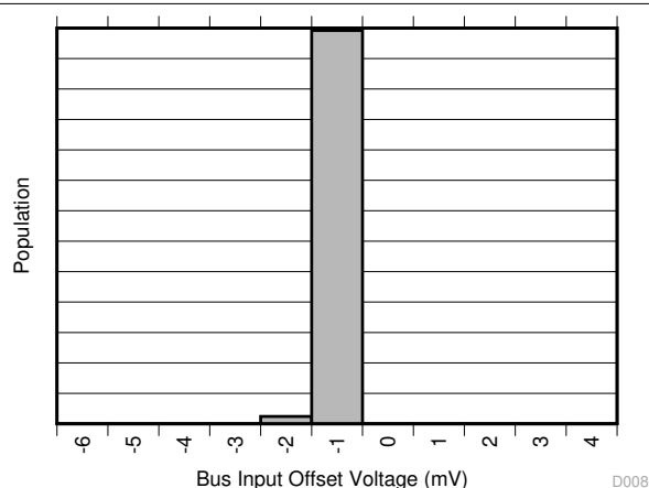
图 5-8. Bus Input Offset Voltage Production Distribution
