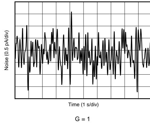
图 26. 0.1-Hz to 10-Hz RTI Current Noise
