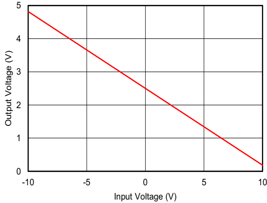
图 9-4. PLC 输出电压与输入电压之间的关系
