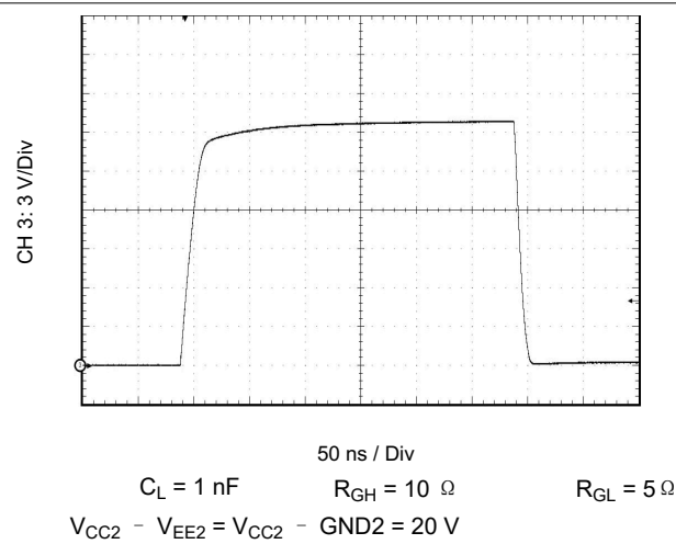
图 7-12. Output Transient Waveform
