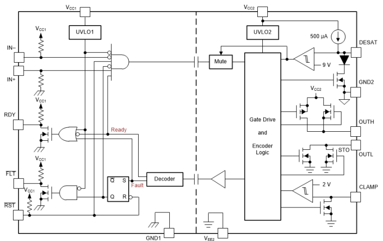
功能方框图
