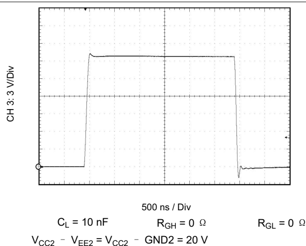
图 7-10. Output Transient Waveform
