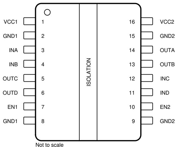
图 4-3. ISO6742-Q1 DWV 封装 16 引脚 SOIC-Extra-WB、SOIC-WB 顶视图
