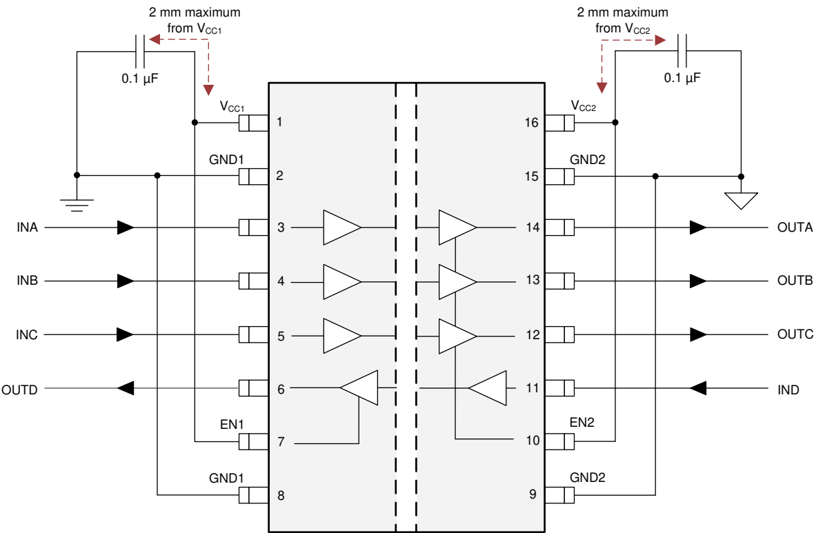
图 8-2. 典型 ISO674x-Q1 电路连接
