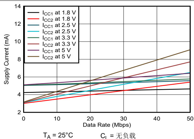
图 5-4. ISO6760-Q1 电源电流与数据速率间的关系 (无负载)
