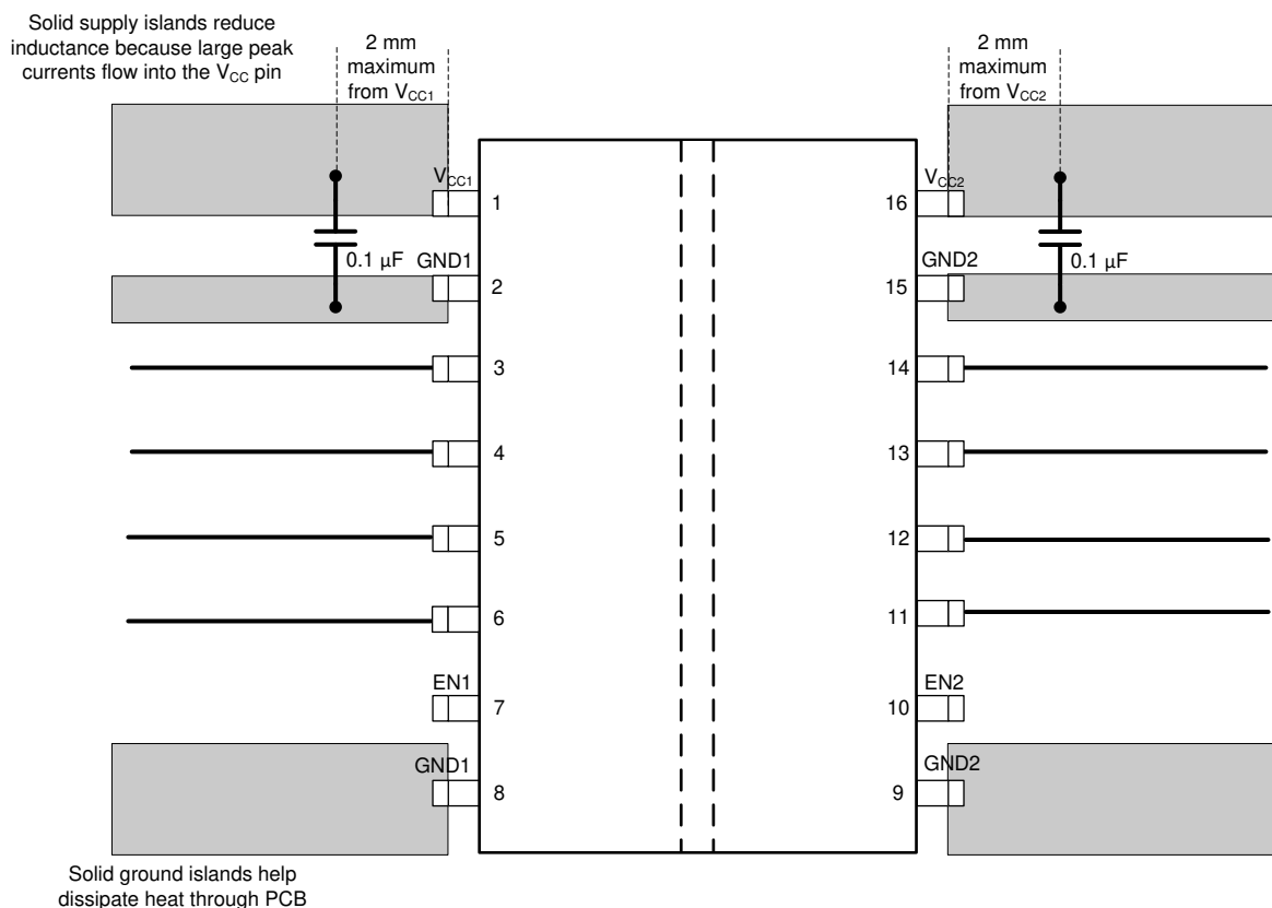
图 8-9. 布局示例
