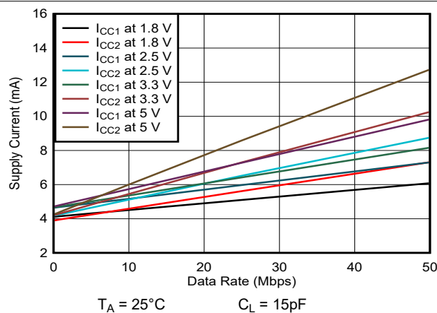
图 5-7. ISO6762-Q1 电源电流与数据速率间的关系 (具有 15pF 负载)
