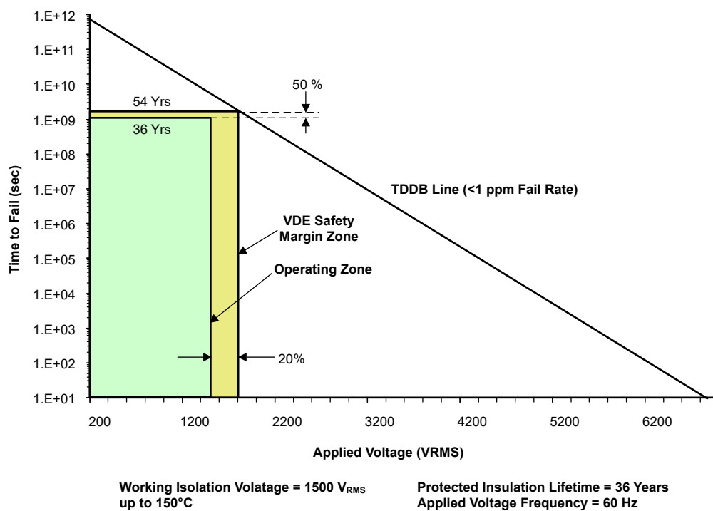
图 8-8. 绝缘寿命预测数据
