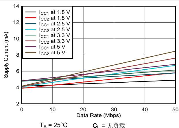
图 5-6. ISO6761-Q1 电源电流与数据速率间的关系 (无负载)
