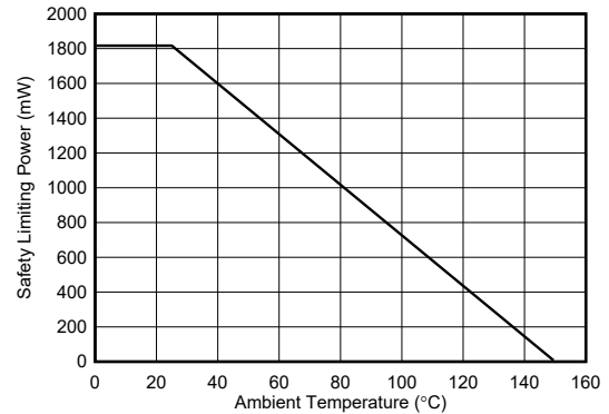
图 5-2. DW-16 封装安全限制功率的热降额曲线
