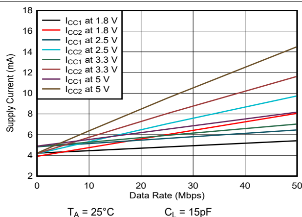
图 5-5. ISO6761-Q1 电源电流与数据速率间的关系 (具有 15pF 负载)
