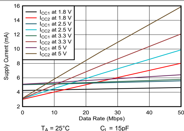
图 5-3. ISO6760-Q1 电源电流与数据速率间的关系 (具有 15pF 负载)
