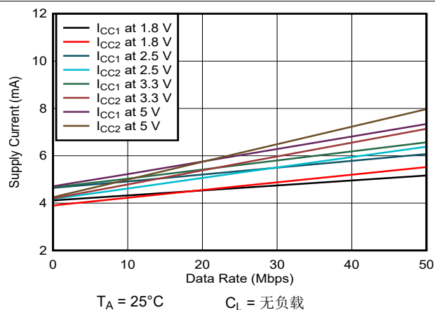
图 5-8. ISO6762-Q1 电源电流与数据速率间的关系 (无负载)
